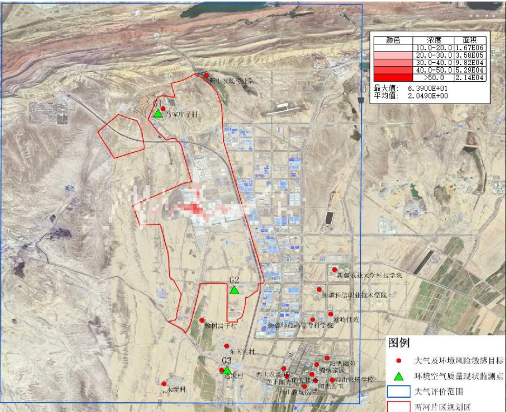
图 5.2-19 二甲苯 1 小时平均最大落地浓度叠加现状值等值线浓度图
