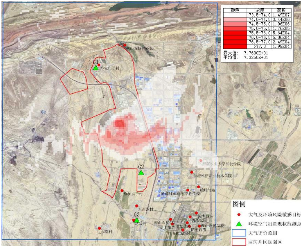
图 5.2-8 PM 10 年平均最大落地浓度叠加现状值等值线浓度图
