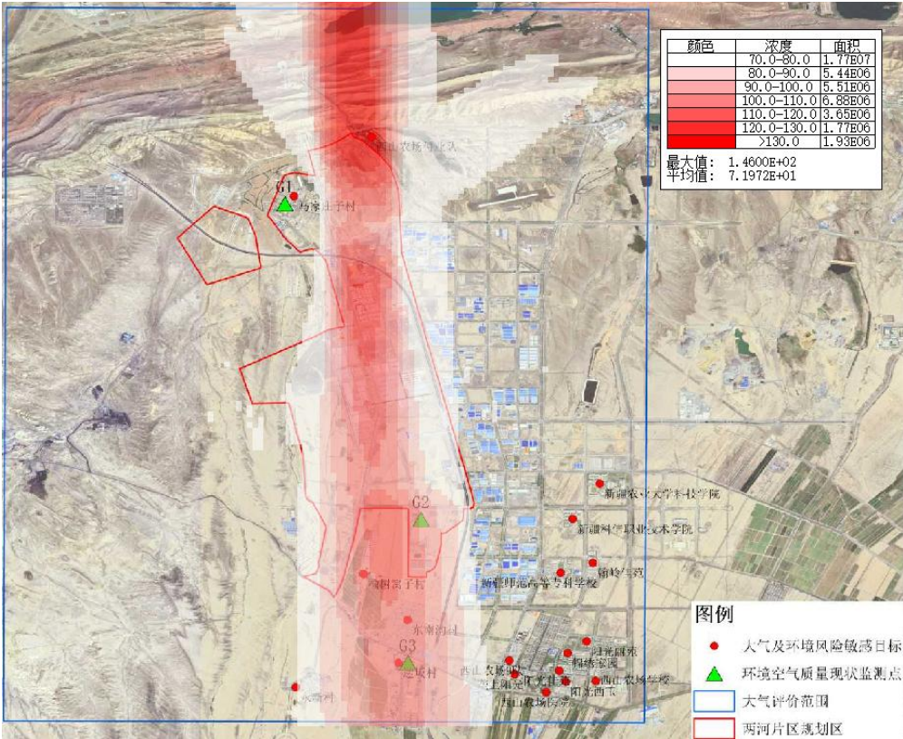
图 5.2-29 氨气 1 小时平均最大落地浓度叠加现状值等值线浓度图
