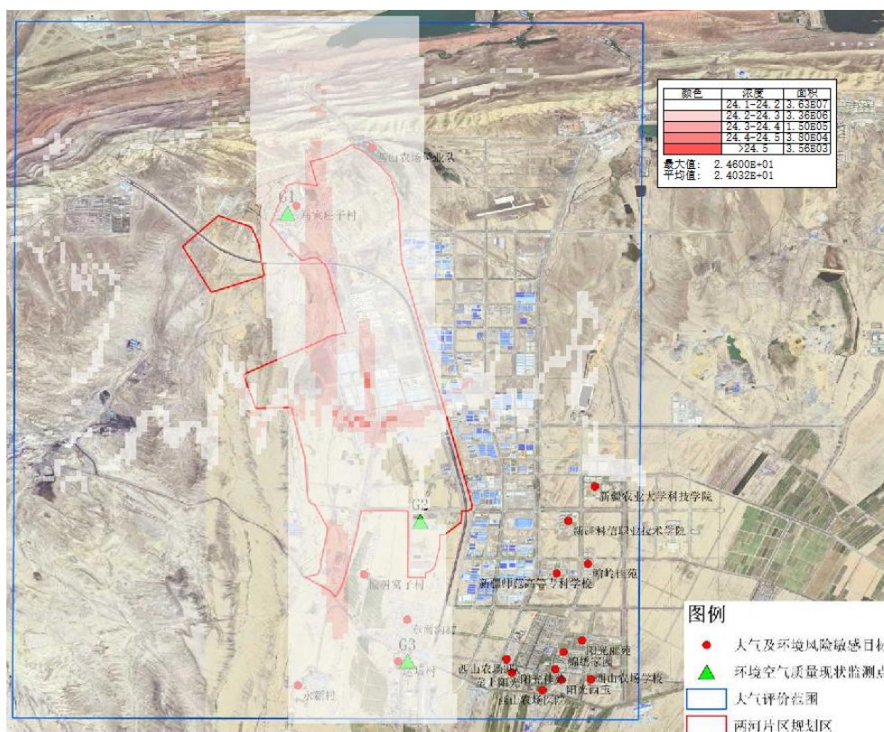
图 5.2-27 氯化氢 1 小时最大落地浓度叠加现状值等值线浓度图
