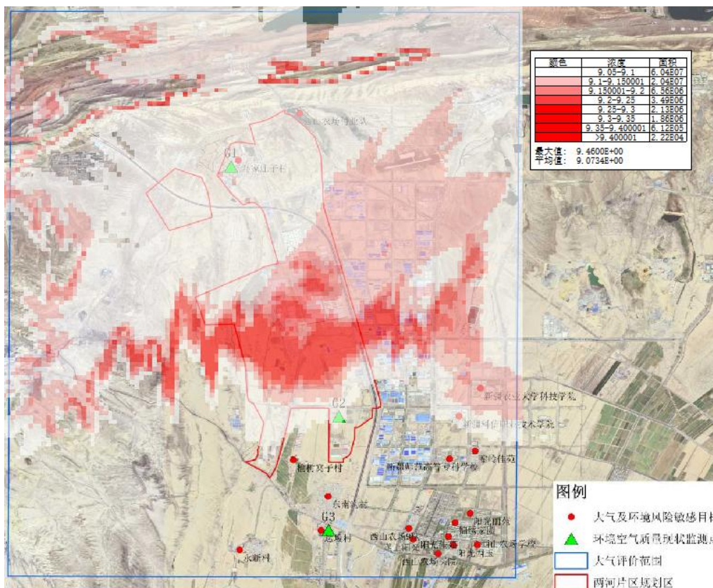
图 5.2-11 SO 2 98%保证率下 24h 平均最大落地浓度叠加现状值等值线浓度图
