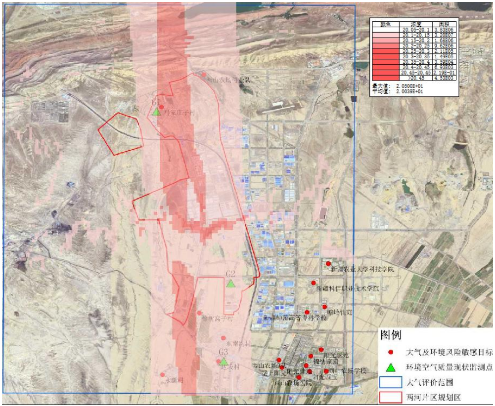
图5.2-31 硫酸雾1小时平均最大落地浓度叠加现状值等值线浓度图
