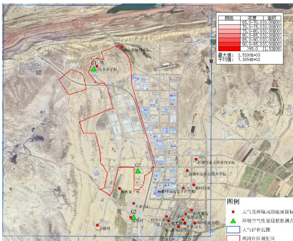
图 5.2-14 非甲烷总烃 1 小时平均最大落地浓度叠加现状值等值线浓度图
