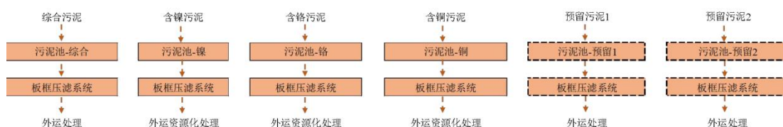
图 3.7-4 污泥处理工艺流程示意图
