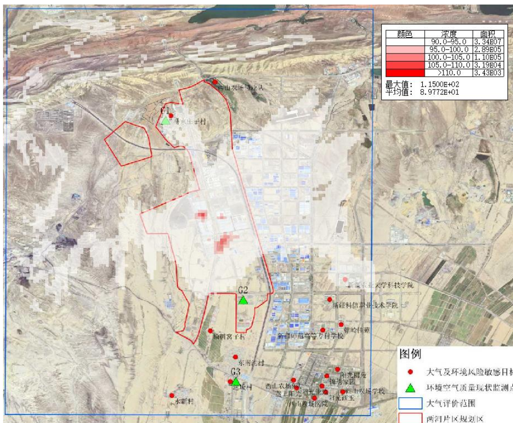
图 5.2-26 NO 2 98%保证率下 24h 平均最大落地浓度叠加现状值等值线浓度图
