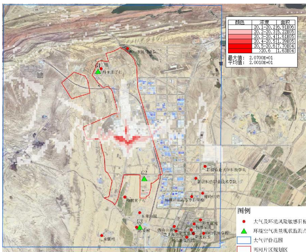
图 5.2-18 硫酸雾 1 小时平均最大落地浓度叠加现状值等值线浓度图
