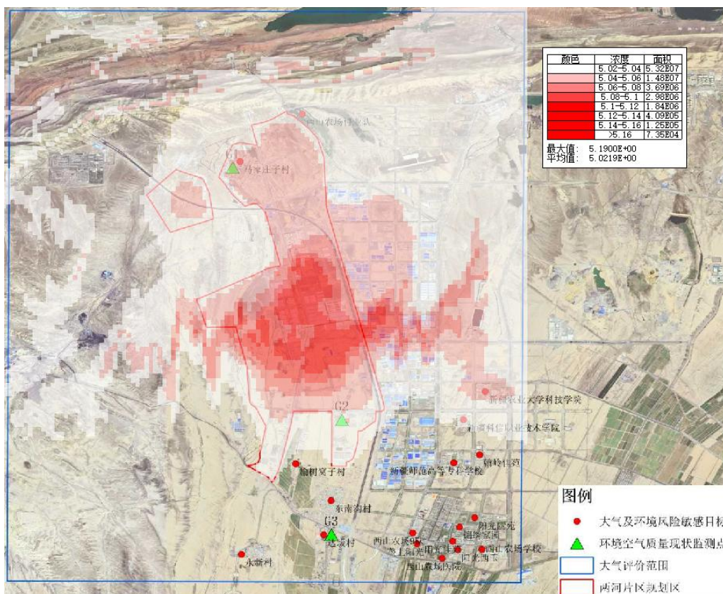
图 5.2-25 SO 2 年平均最大落地浓度叠加现状值等值线浓度图
