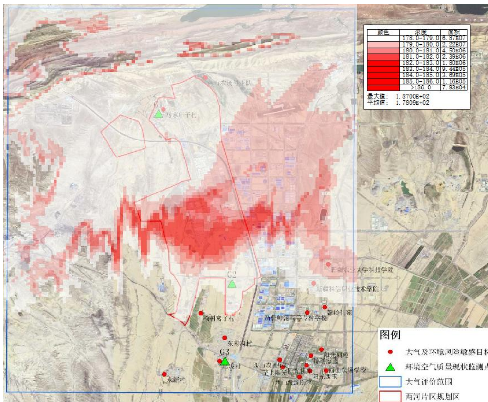
图 5.2-20 PM 10 95%保证率下 24h 平均最大落地浓度叠加现状值等值线浓度图
