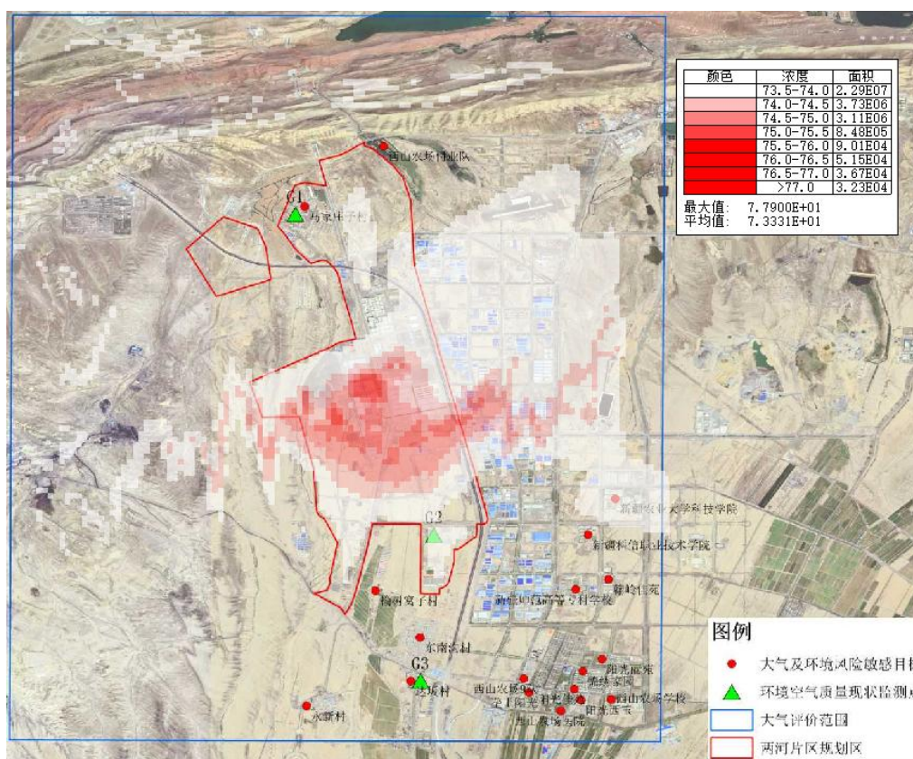
图 5.2-21 PM 10 年平均最大落地浓度叠加现状值等值线浓度图
