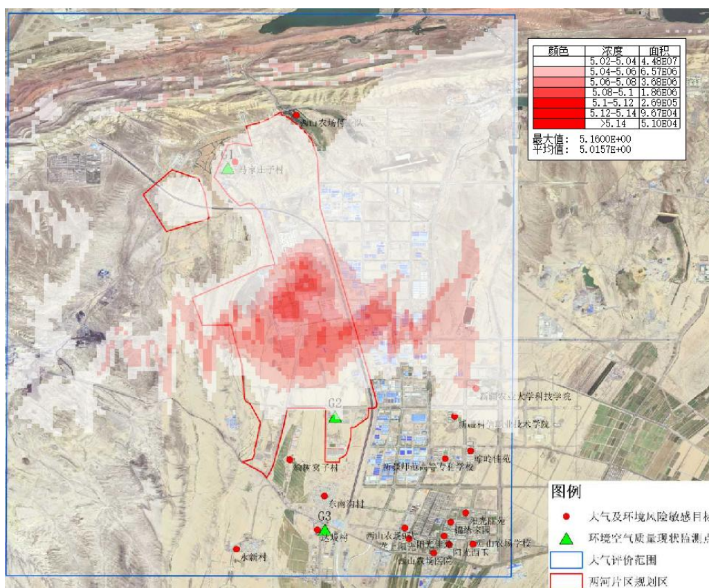
图 5.2-12 SO 2 年平均最大落地浓度叠加现状值等值线浓度图
