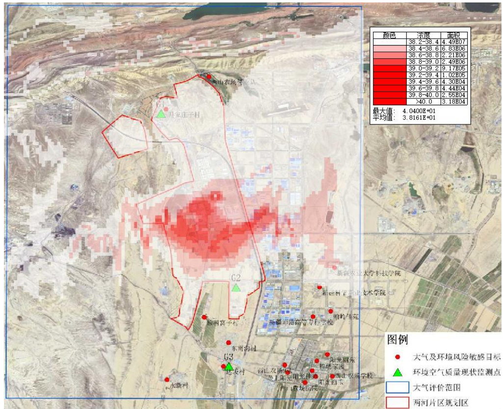
图 5.2-23 PM 2.5 年平均最大落地浓度叠加现状值等值线浓度图
