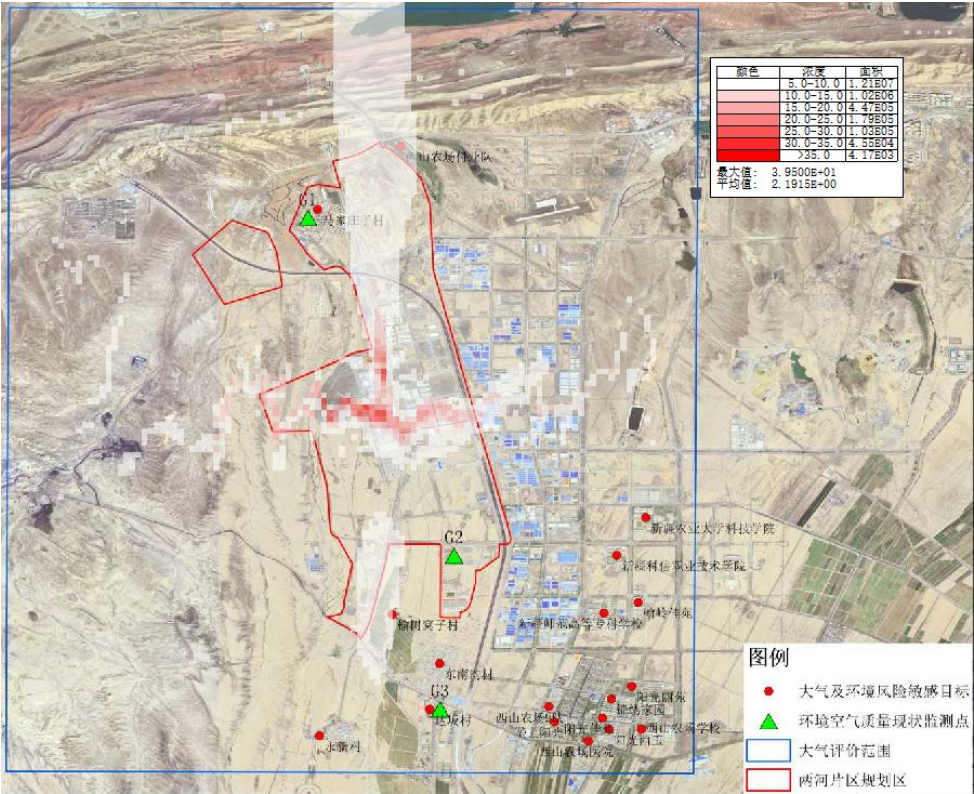
图 5.2-28 二甲苯 1 小时平均最大落地浓度叠加现状值等值线浓度图
