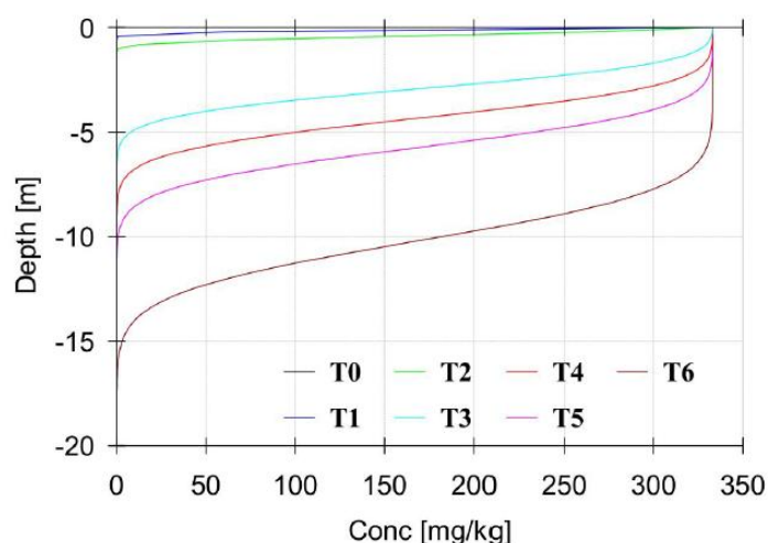
图 5.7-3 土壤中氰化物渗漏预测结果
