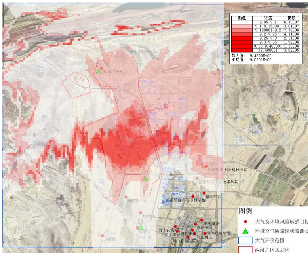
图 5.2-24 SO 2 98%保证率下 24h 平均最大落地浓度叠加现状值等值线浓度图
