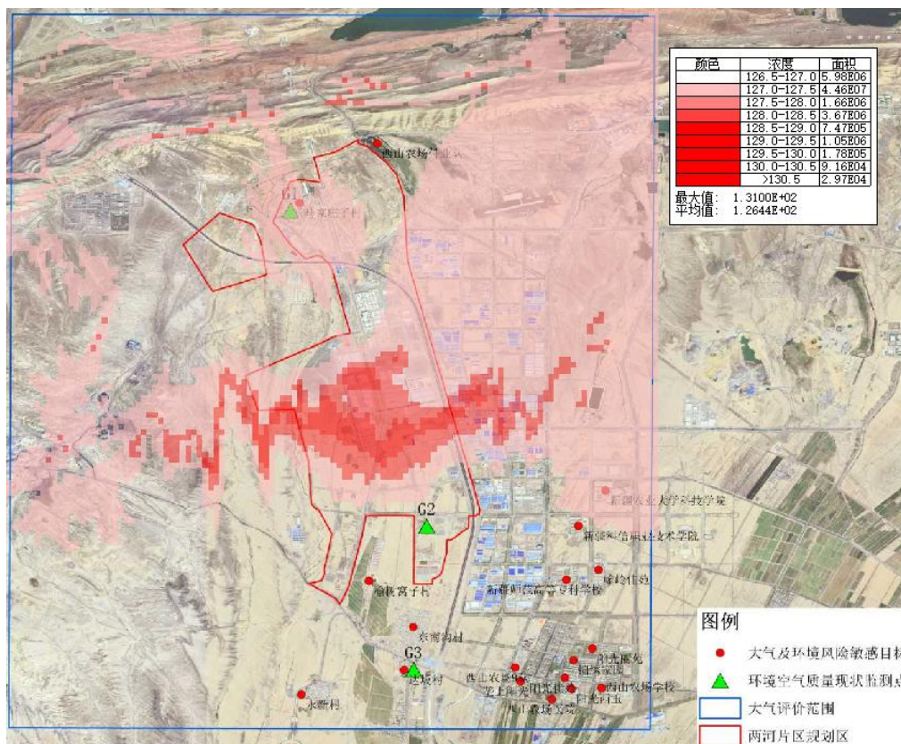
图 5.2-9 PM 2.5 95%保证率下 24h 平均最大落地浓度叠加现状值等值线浓度图
