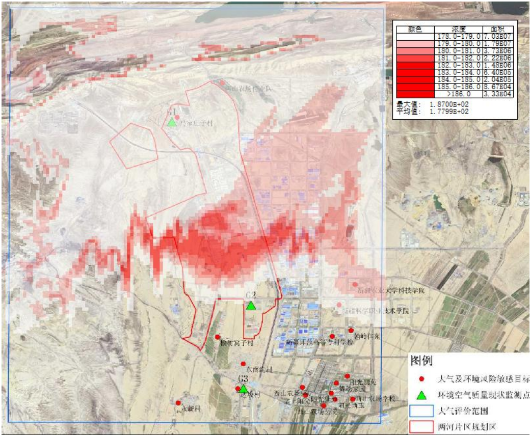
图 5.2-7 PM 10 95%保证率下 24h 平均最大落地浓度叠加现状值等值线浓度图
