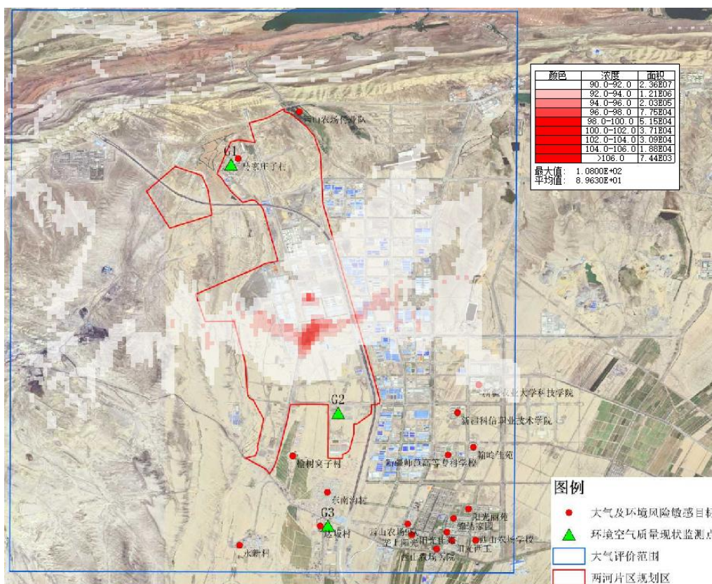
图 5.2-13 NO 2 98%保证率下 24h 平均最大落地浓度叠加现状值等值线浓度图
