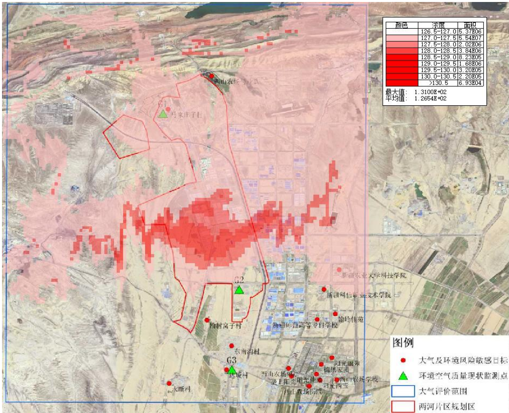
图 5.2-22 PM 2.5 98%保证率下 24h 平均最大落地浓度叠加现状值等值线浓度图
