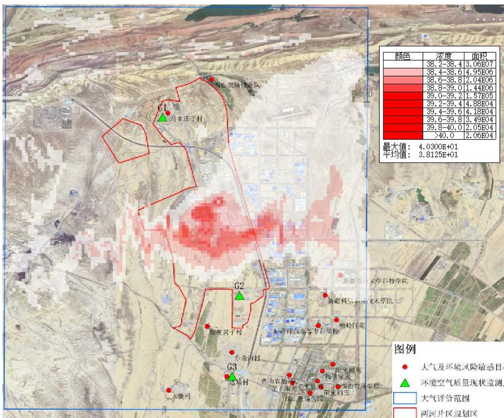
图 5.2-10 PM 2.5 年平均最大落地浓度叠加现状值等值线浓度图
