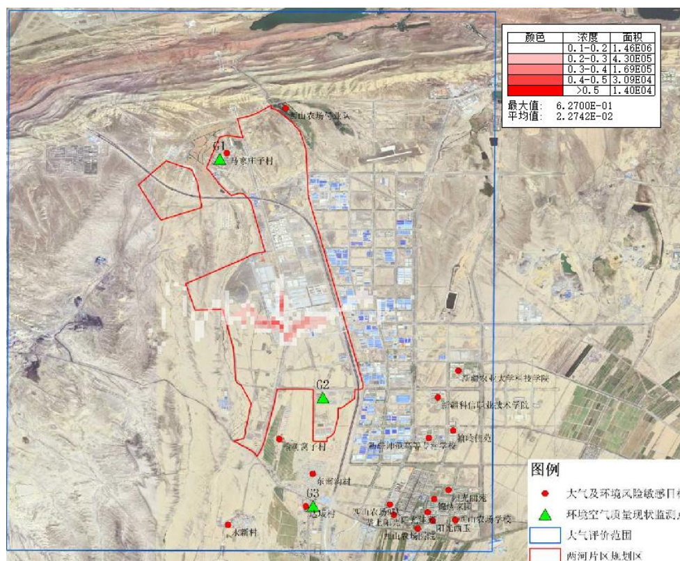
图 5.2-16 硫化氢 1 小时平均最大落地浓度叠加现状值等值线浓度图
