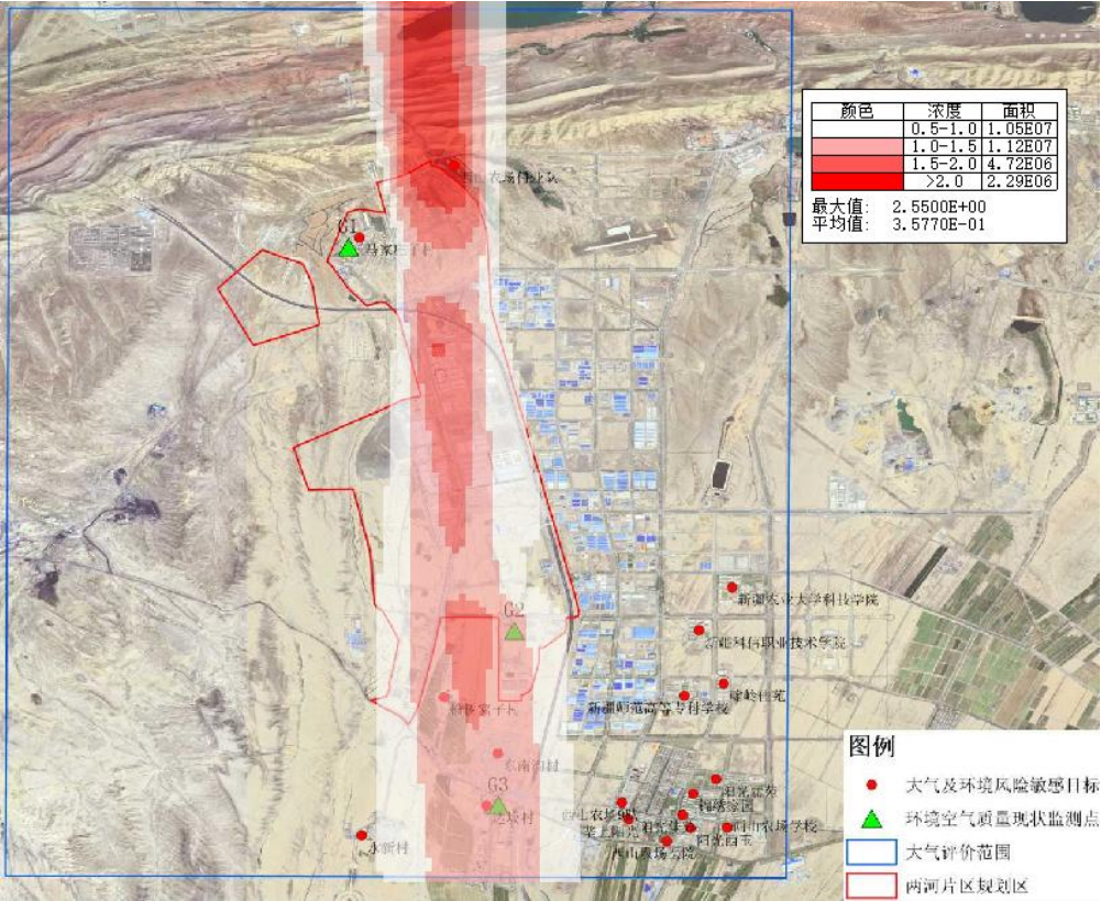
图 5.2-30 硫化氢 1 小时平均最大落地浓度叠加现状值等值线浓度图
