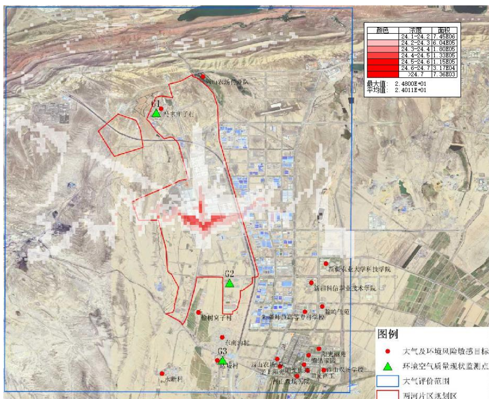
图 5.2-17 氯化氢 1 小时平均最大落地浓度叠加现状值等值线浓度图
