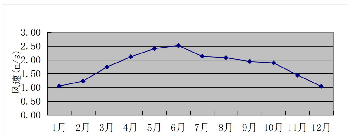
图 5.2-3 年平均风速月变化曲线
