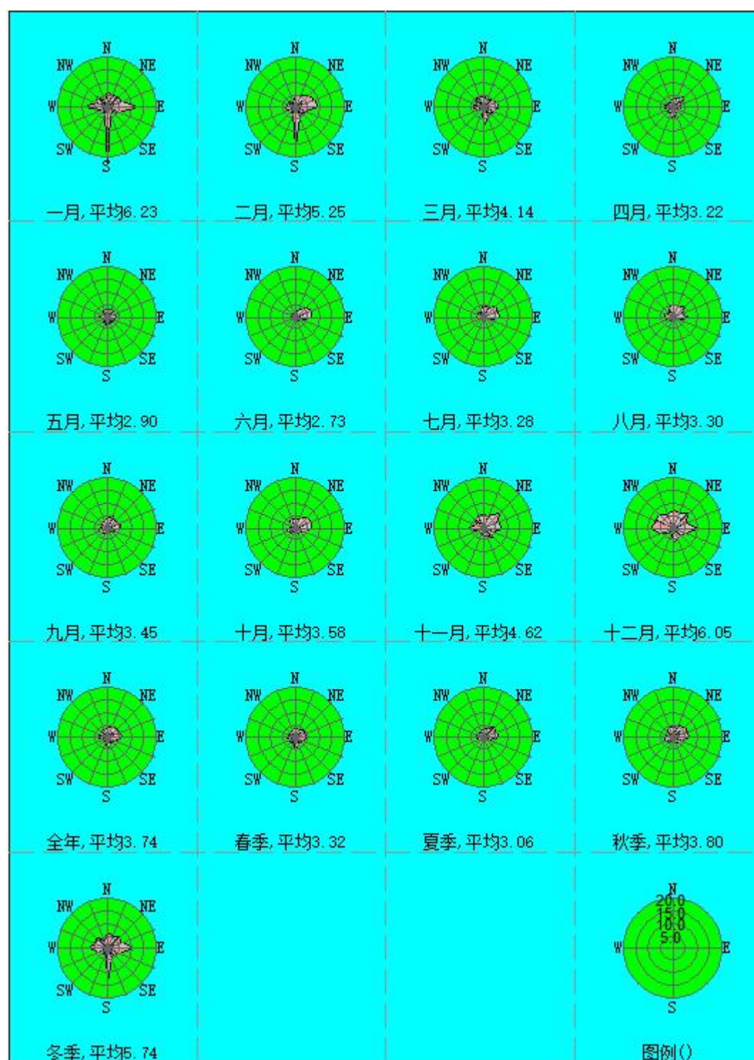
图 5.2-6 2024 年全年和各季污染系数玫瑰图
