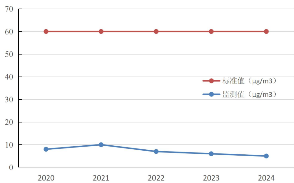
图 3.3-1 2020~2024 年 SO 2 变化趋势图
