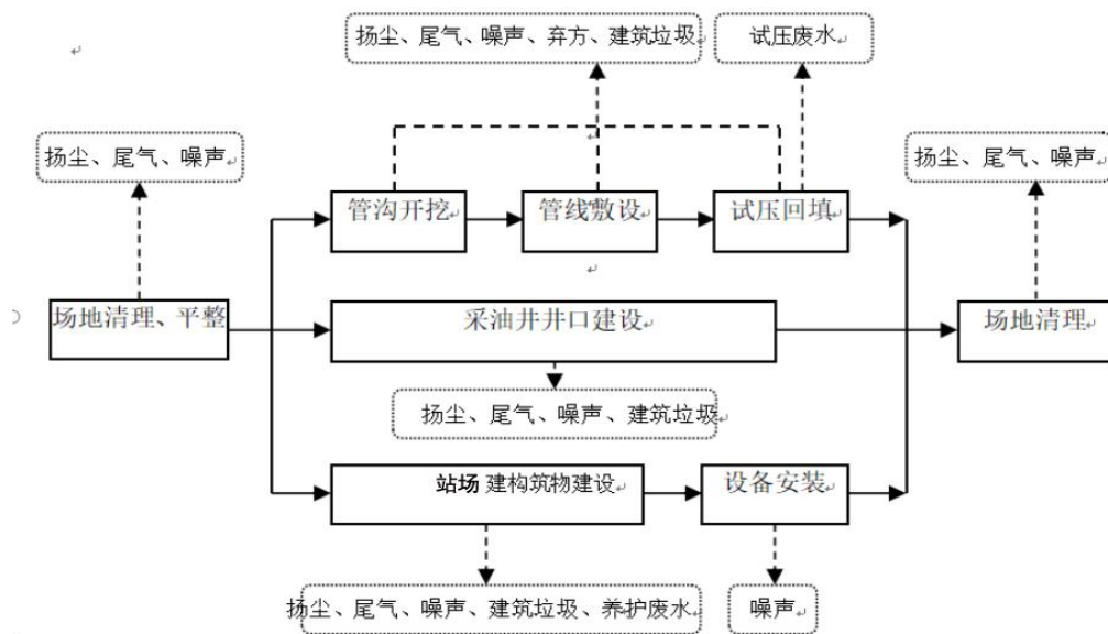
图 3.4-1 井场和站场建设流程及产污环节示意图
