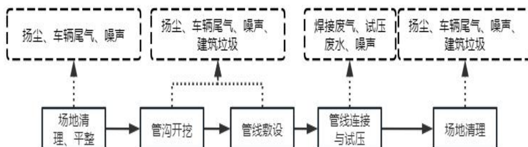
图 3.4-2 管道工程施工阶段工艺流程图
