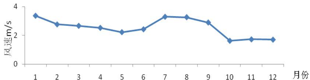
图 5.5-1 评价区全年各月风速变化曲线
