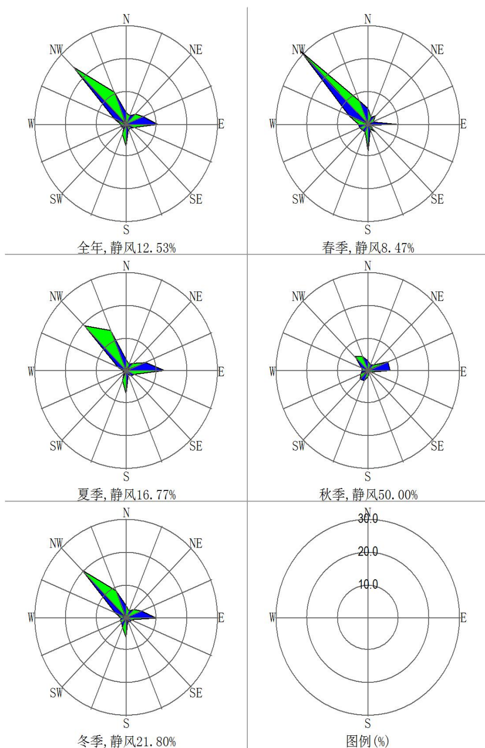
图 5.2-2 克拉玛依市全年及各季风向频率玫瑰图
