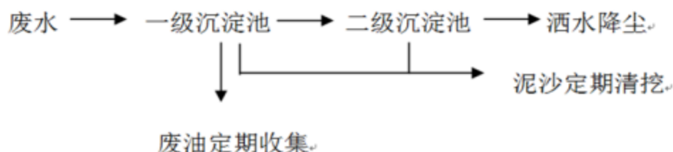
图 6.1-2 机械冲洗废水处理工艺流程图
