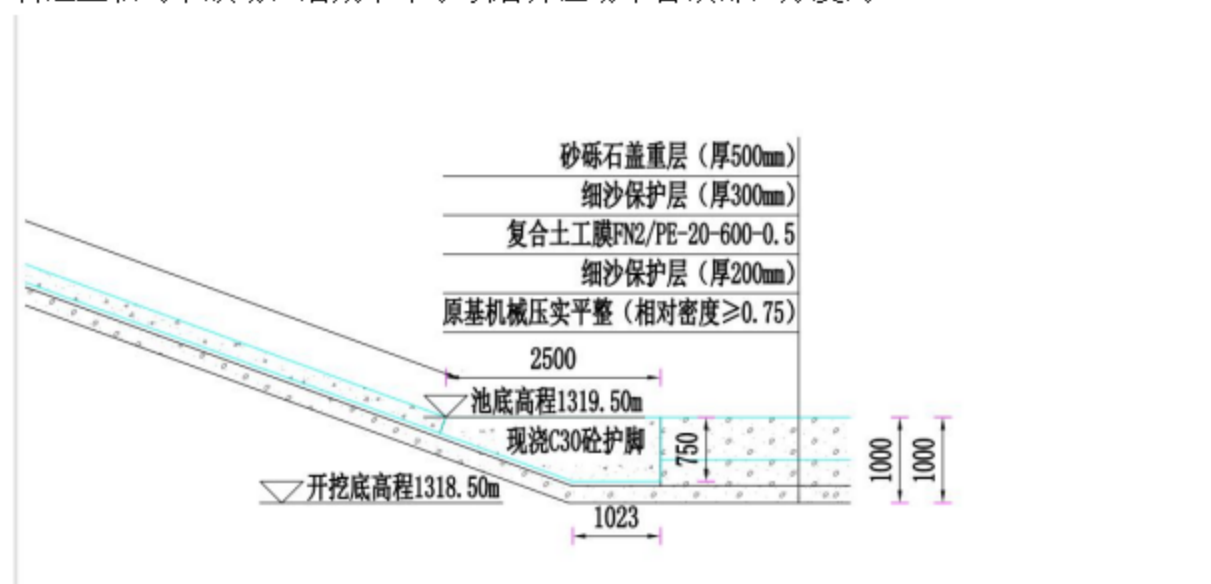
图 3.5-1 库盘开挖示意图
