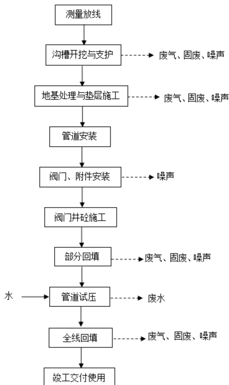
图 3.5-2 输水管道施工工艺流程及产污环节图
