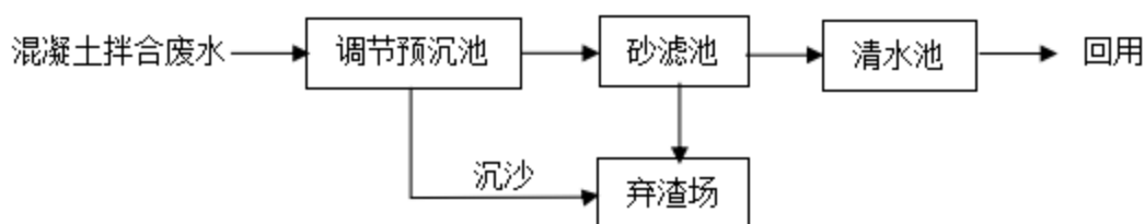
图 6.1-1 混凝土搅拌站废水处理工艺流程示意图
