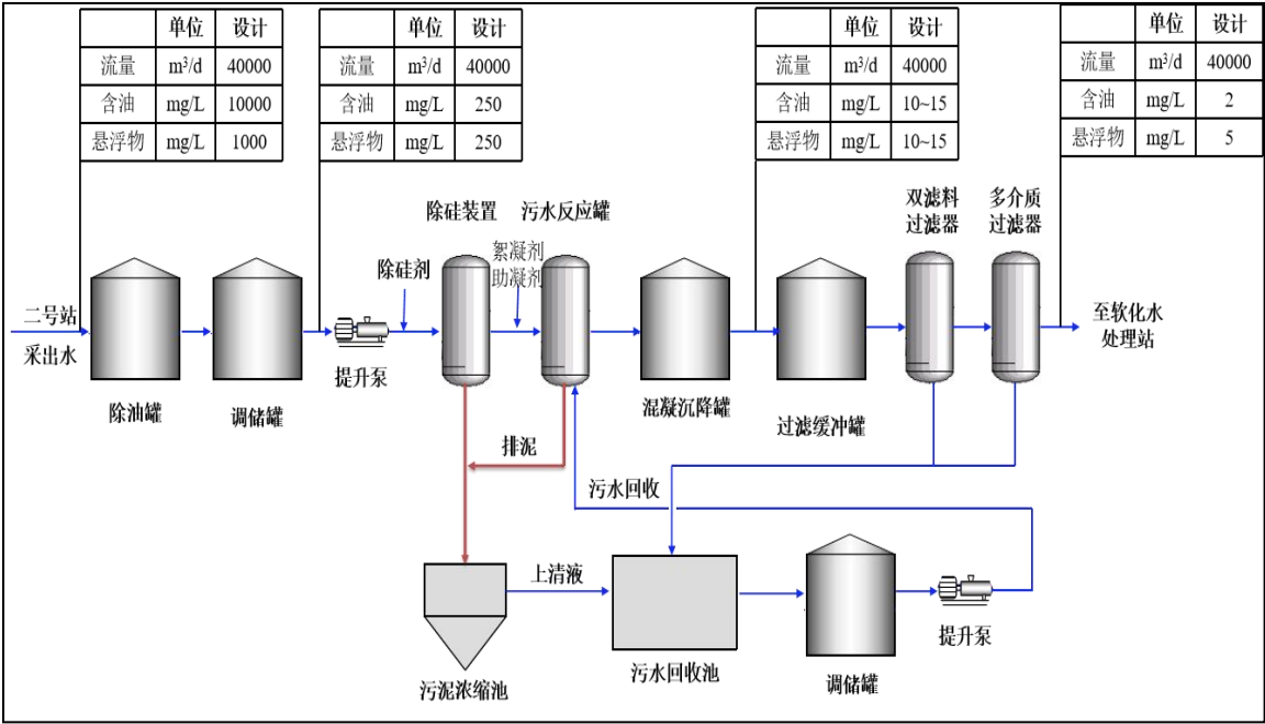
图 3.3-13 风城 2 号稠油联合站采出水水处理流程图
