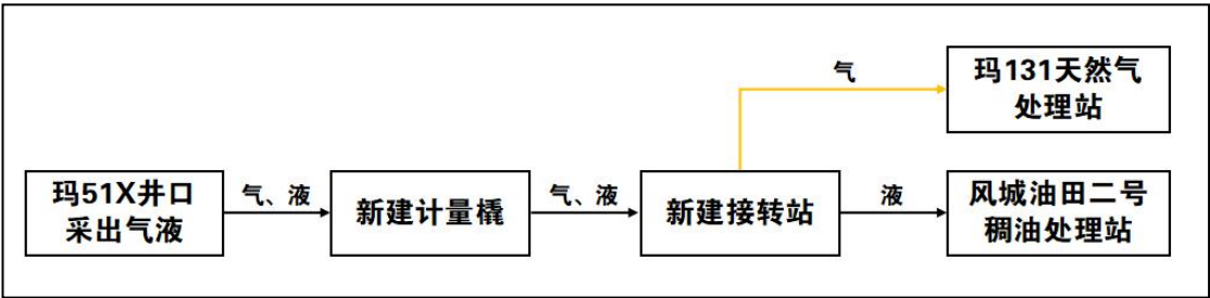
图3.3-2 本项目集输总体流向示意图
