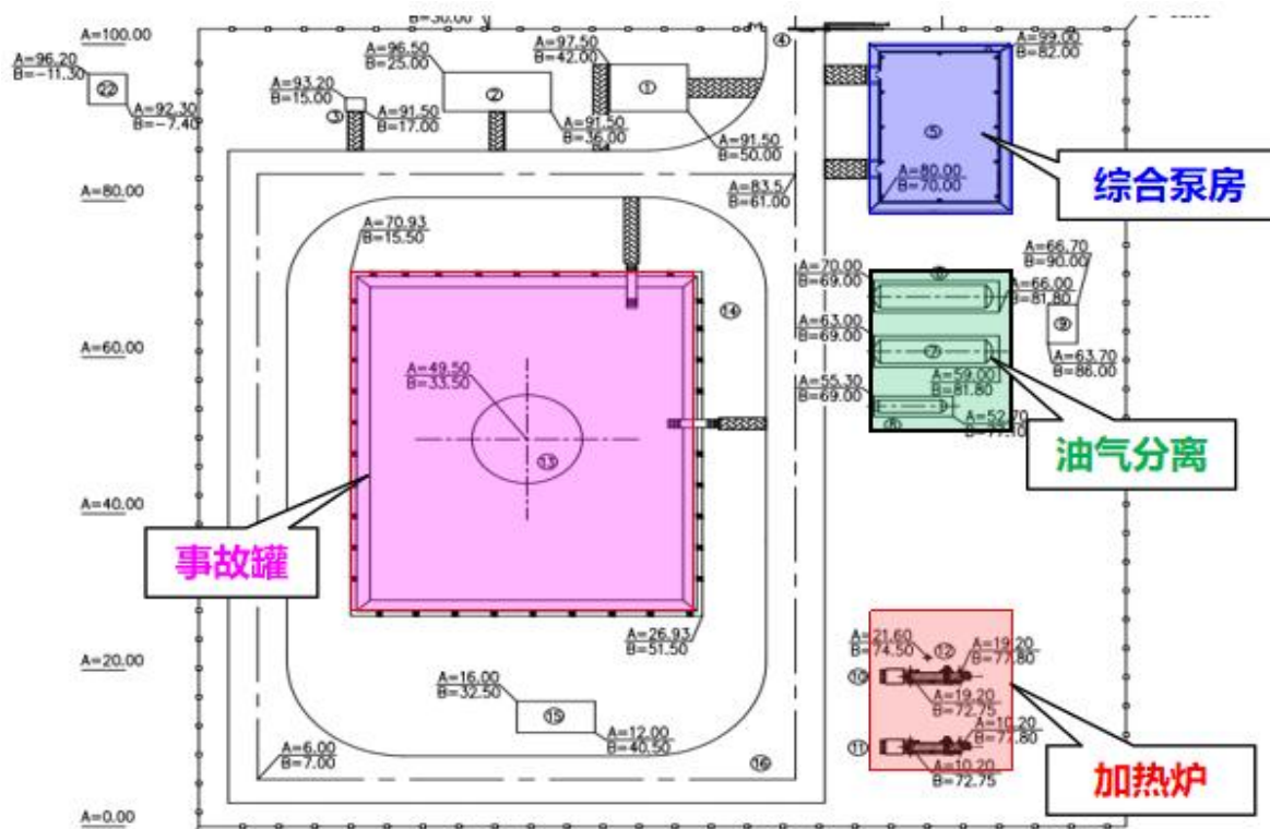
图 3.3-9 转油站平面布置图
