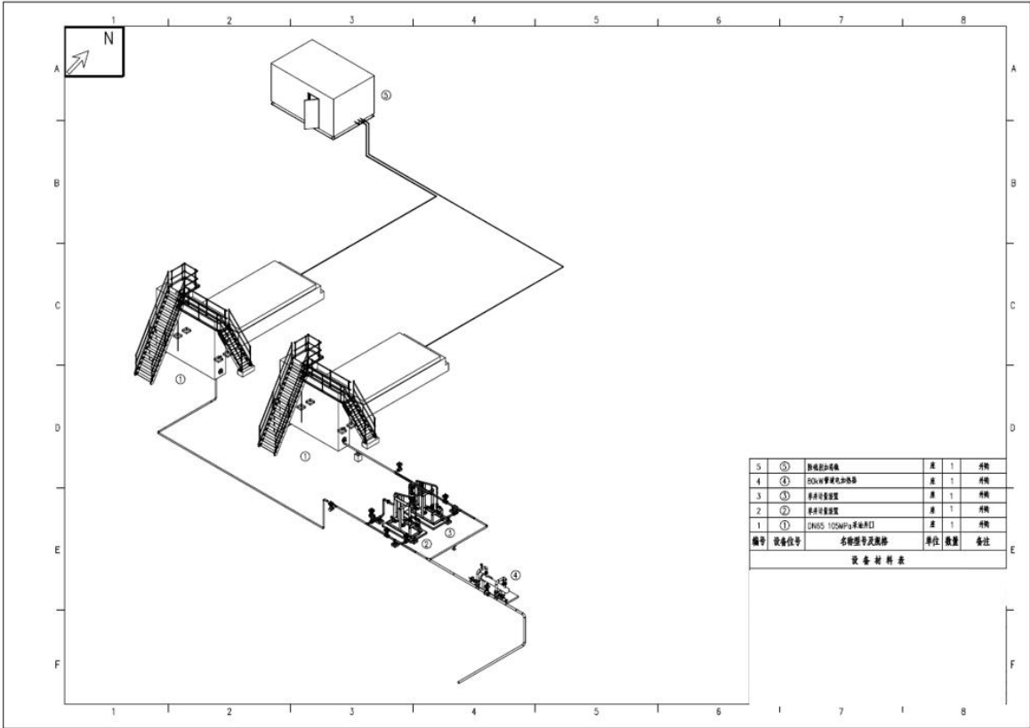
图 3.3-6 平台井平面布置图
