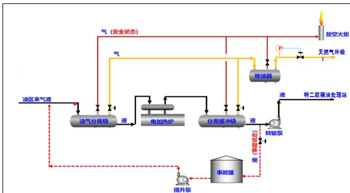
图 3.3-8 玛 51X 转油站工艺流程图
