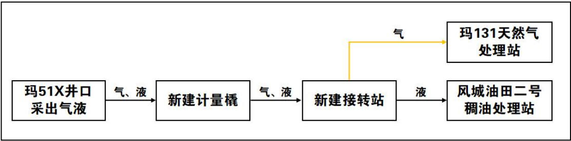
图3.3-10 油区集输工艺流程图
