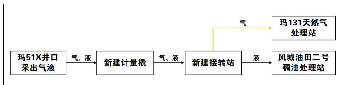
图 3.4-7 本项目工艺流程
