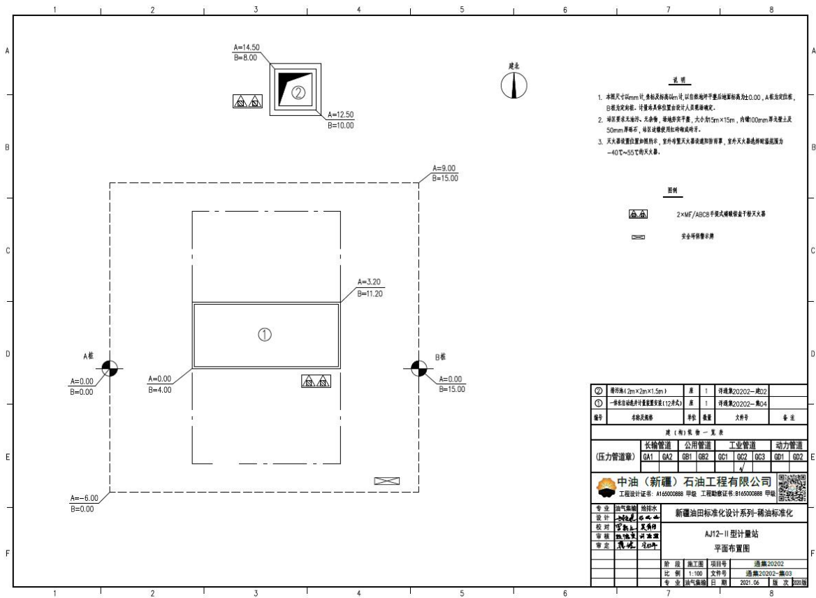
图 3.3-7 计量站平面布置图
