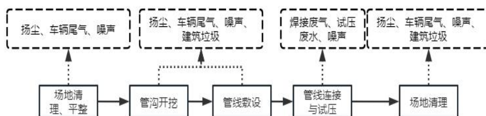
图 3.4-5 管道工程施工阶段工艺流程图
