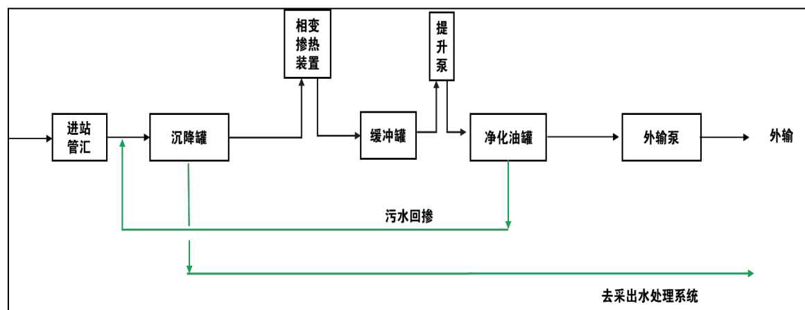
图 3.3-12 风城 2 号稠油联合站原油处理工艺流程示意图
