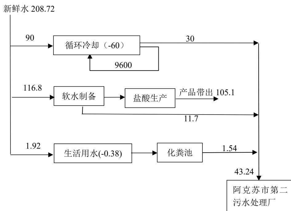
图 3.2-3 项目给排水平衡图 \text{m}^3/\text{d}
