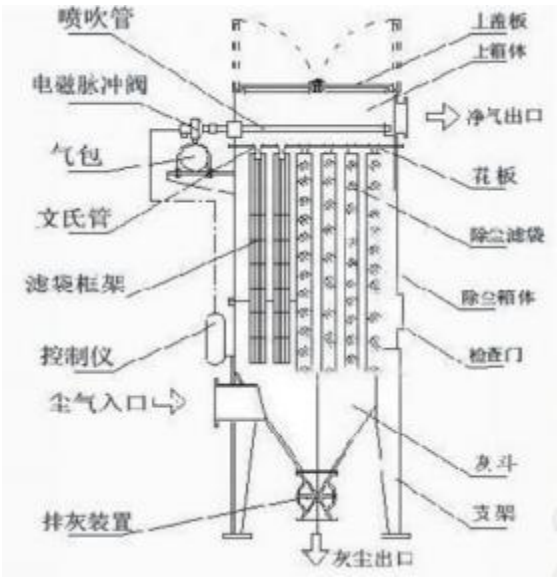
图 6.1-1 脉冲袋式除尘器结构示意图
