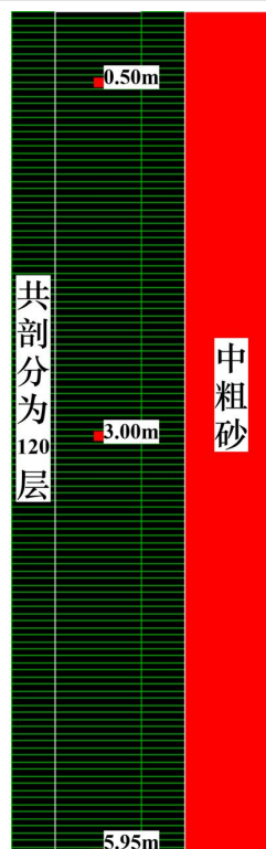
图 5.7-1 土壤岩性概化及观测点分布图
