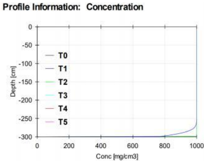
图 5.5-3 不同时刻石油类浓度-剖面深度变化曲线图
