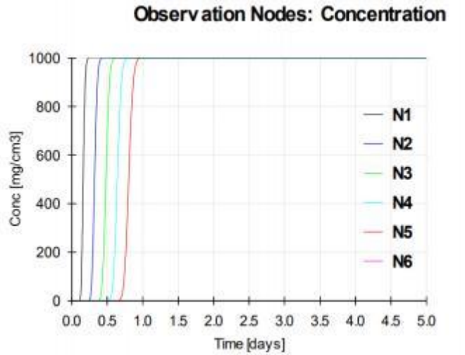
图 5.5-2 不同观测点处石油类浓度-时间变化曲线图
