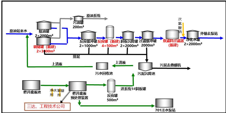
图 2.1-5 81 号集中处理站污水处理系统工艺流程图
