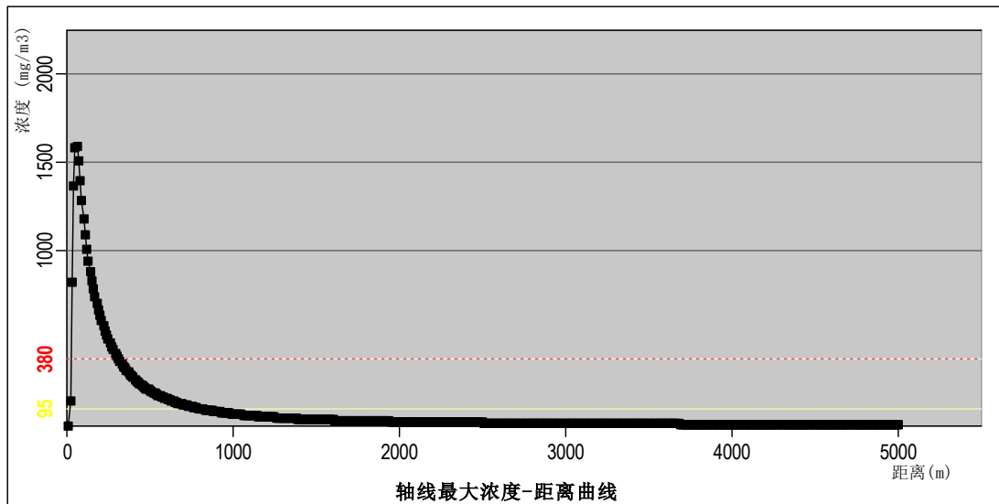
图 1 浓度与扩散距离图
