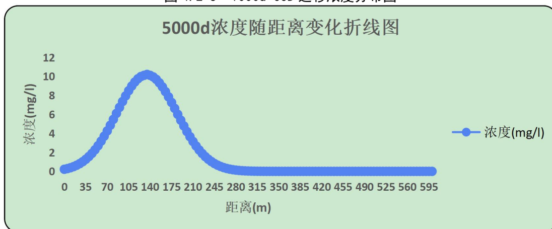
图 4.2-6 5000d COD 运移浓度分布图
