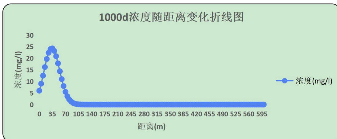
图 4.2-5 1000d COD 运移浓度分布图
