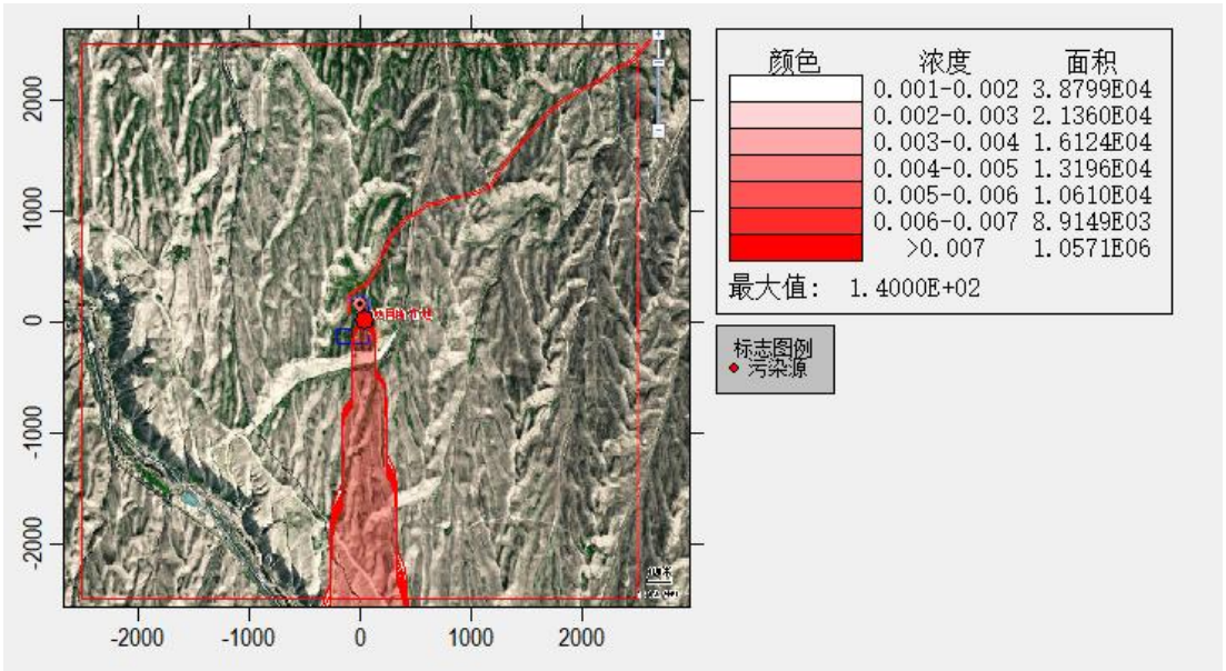
图 2 大气环境风险预测图
