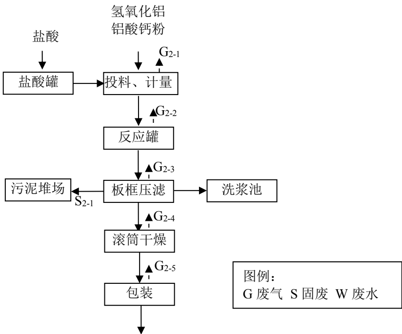
图 3.6-4 饮用水级聚合氯化铝工艺流程图
