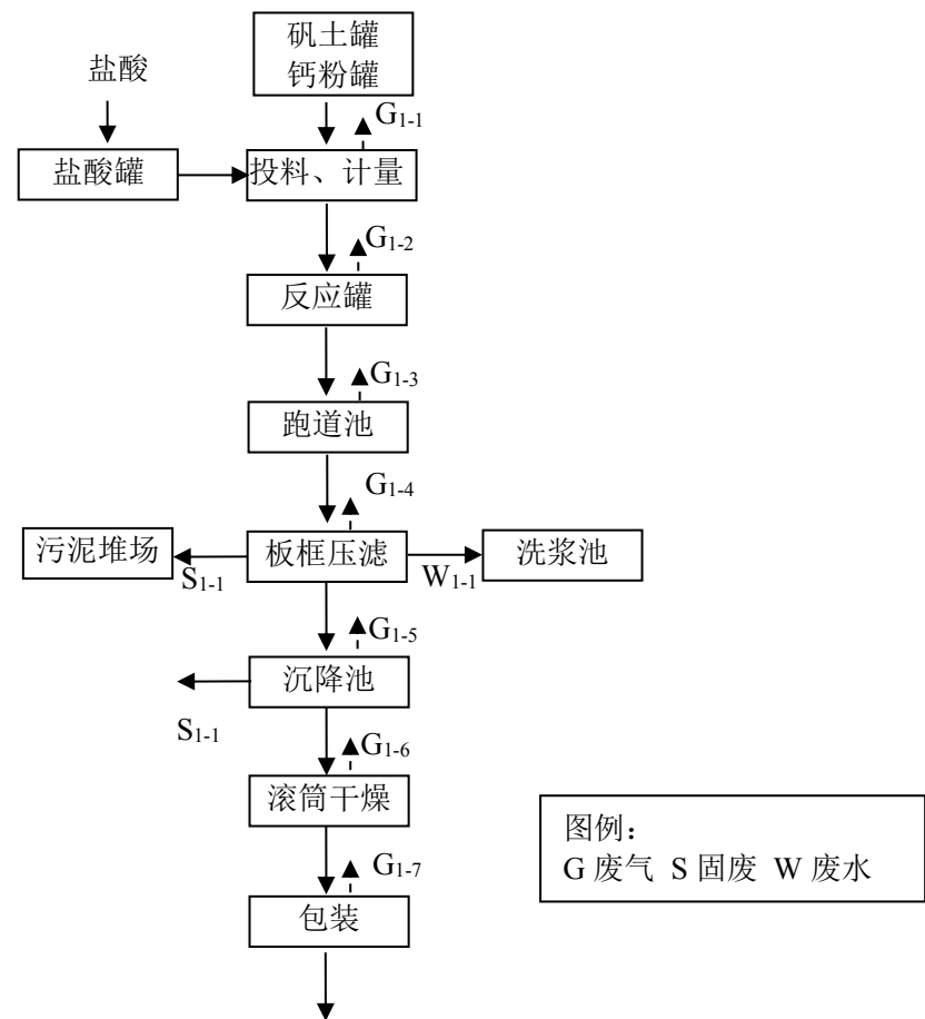
图 3.6-1 工业级聚合氯化铝工艺流程图
