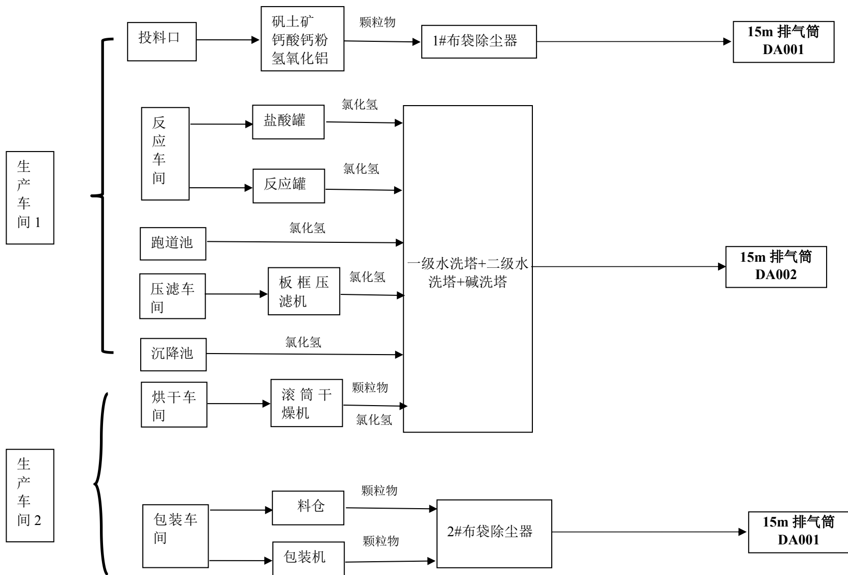
图 3.2.7-1 全厂 90 废气治理示意图
