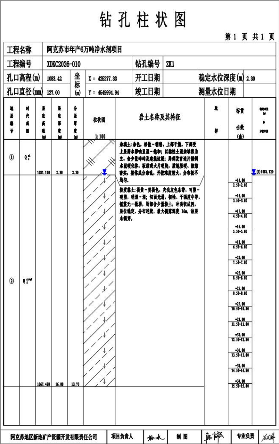
图 5.4-1 厂区钻孔柱状图
