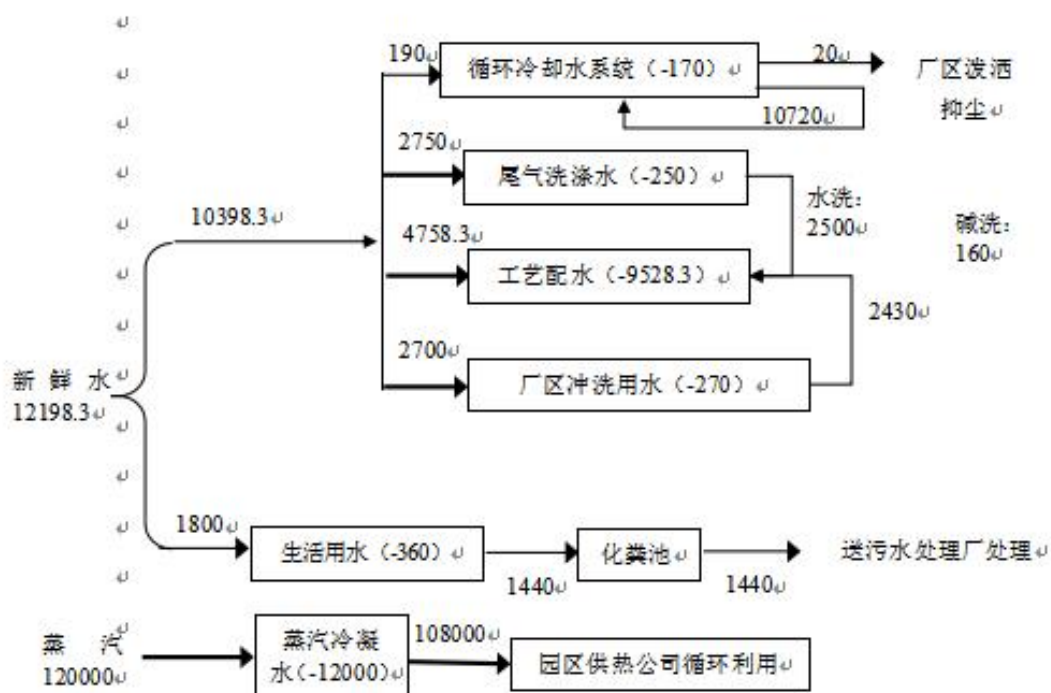
图 3.7-1 全厂给排水平衡图 单位（m³/a）
