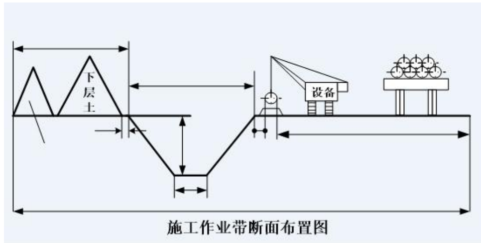
图 3.5-2 一般地段管道施工方式断面示意图
