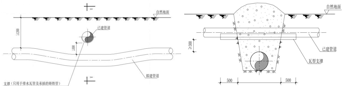
图 3.5-3 管道交叉施工作业示意图
