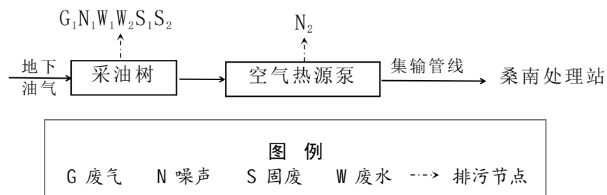
图 3.5-4 轮古 12-H3 井场开采及集输工艺流程图
