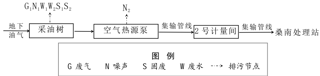
图 3.5-6 轮古 102-1 井场开采及集输工艺流程图
