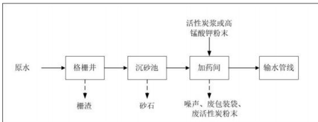
图2.3-5 预处理站工艺及产污节点图
