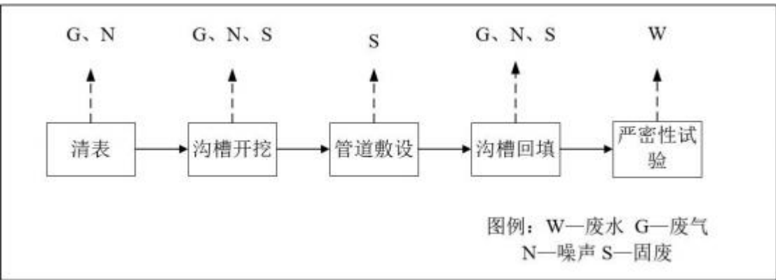
图2.3-2 施工期管道施工（开槽法）工艺及产污节点图
