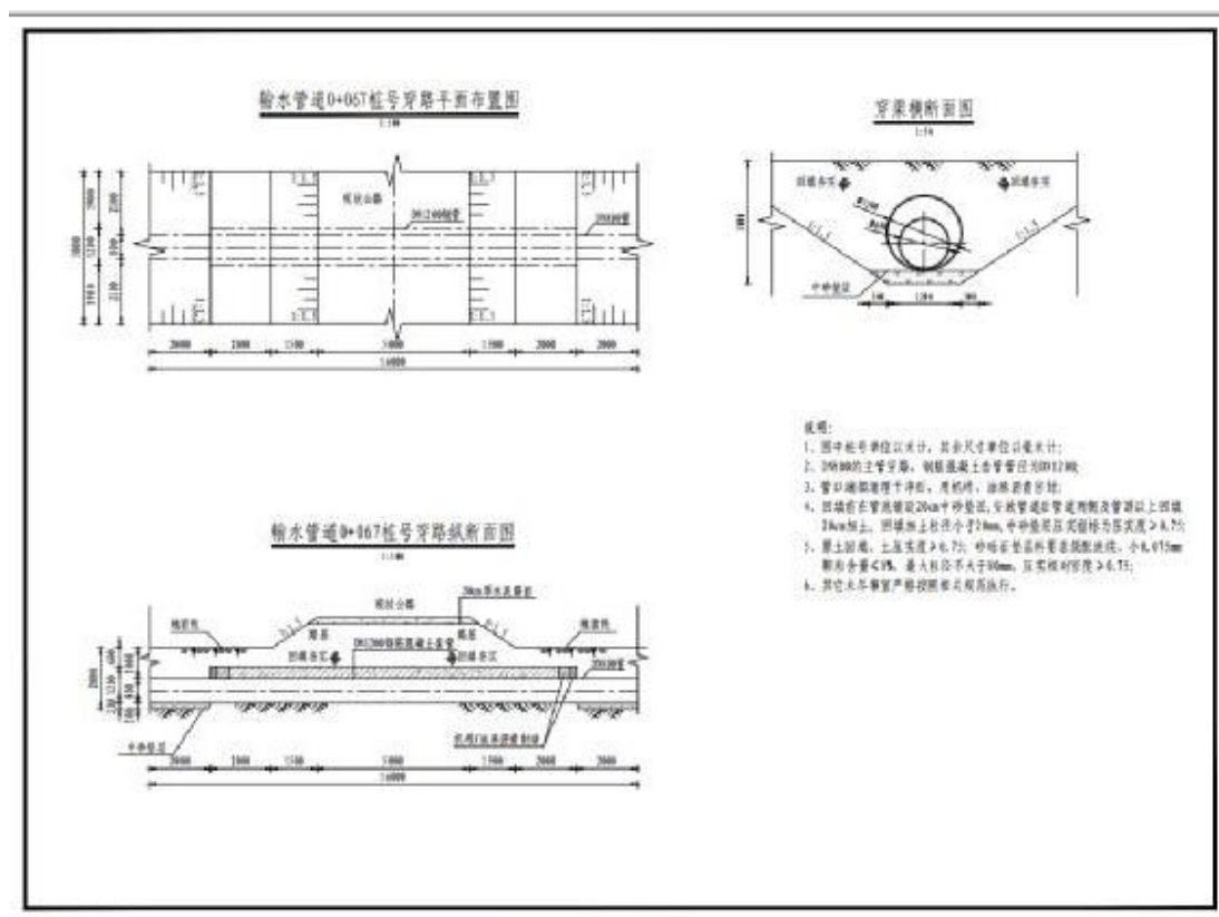
图2.2-2 输水管道穿路平面、纵断面图
