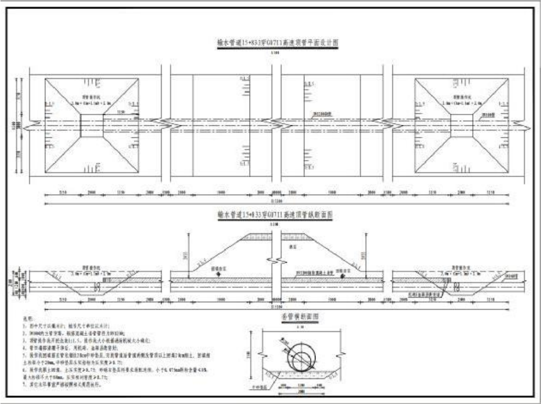
图2.2-1 输水管道穿越高速顶管平面、纵断面图
