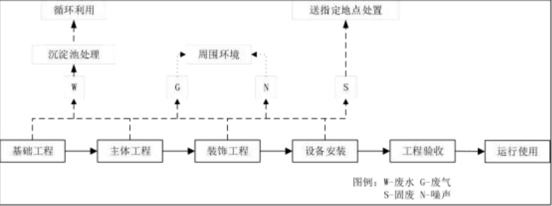
图2.3-1 施工期建筑施工工艺及产污节点图
