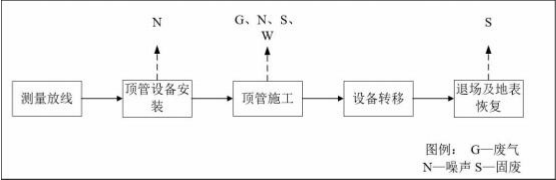
图2.3-4 施工期管道施工（顶管法）工艺及产污节点图
