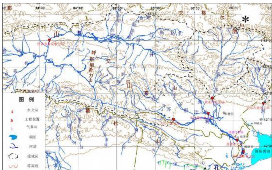
图4.1-4 区域水系图
