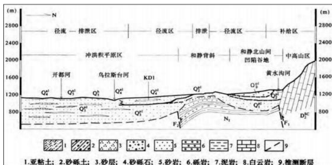
图4.1-3 评价区水文地质剖面图
