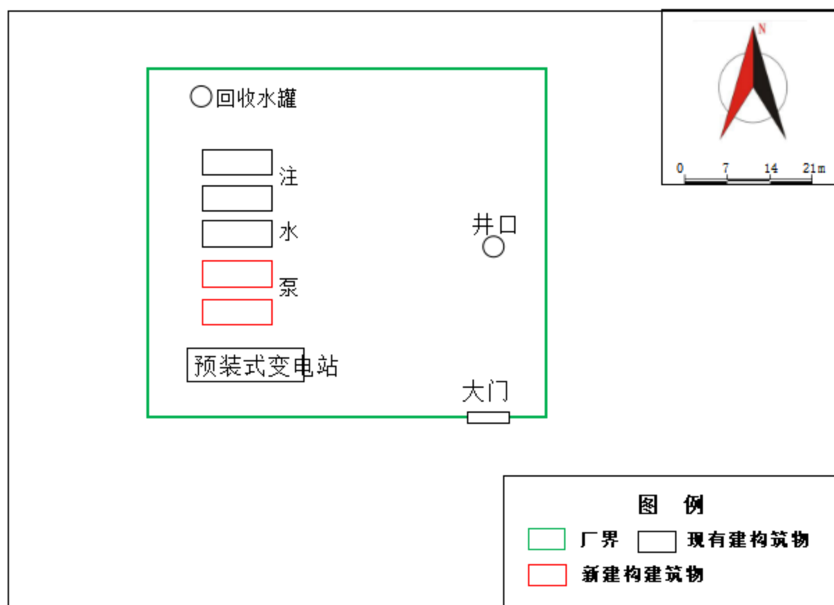
图 3.3-1 轮古 4C 井场运营期平面布置示意图
