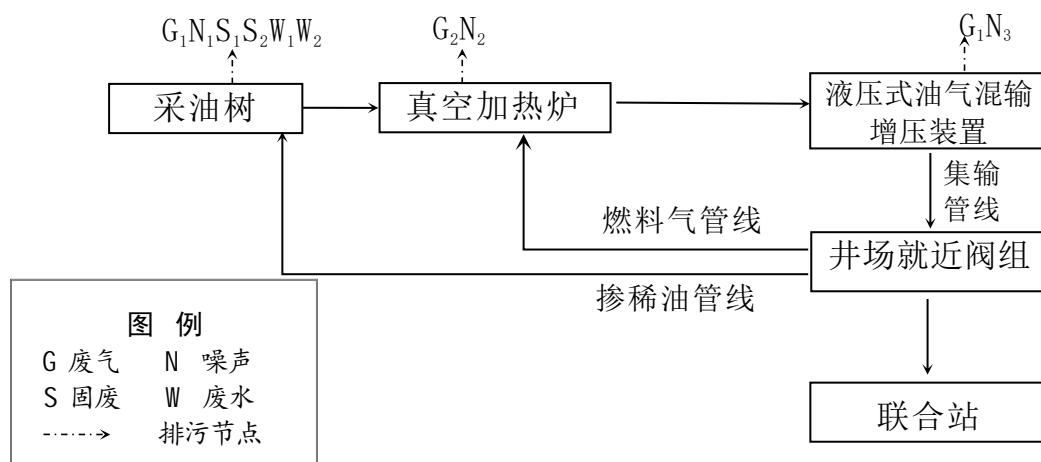
图 3.3-5 YQ9-6 井场工艺流程图
