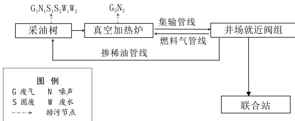
图 3.3-5 YQ9-6 井场工艺流程图
