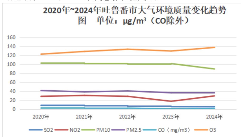
图 3.4.1-2 2020~2024 年常规因子浓度变化趋势图
