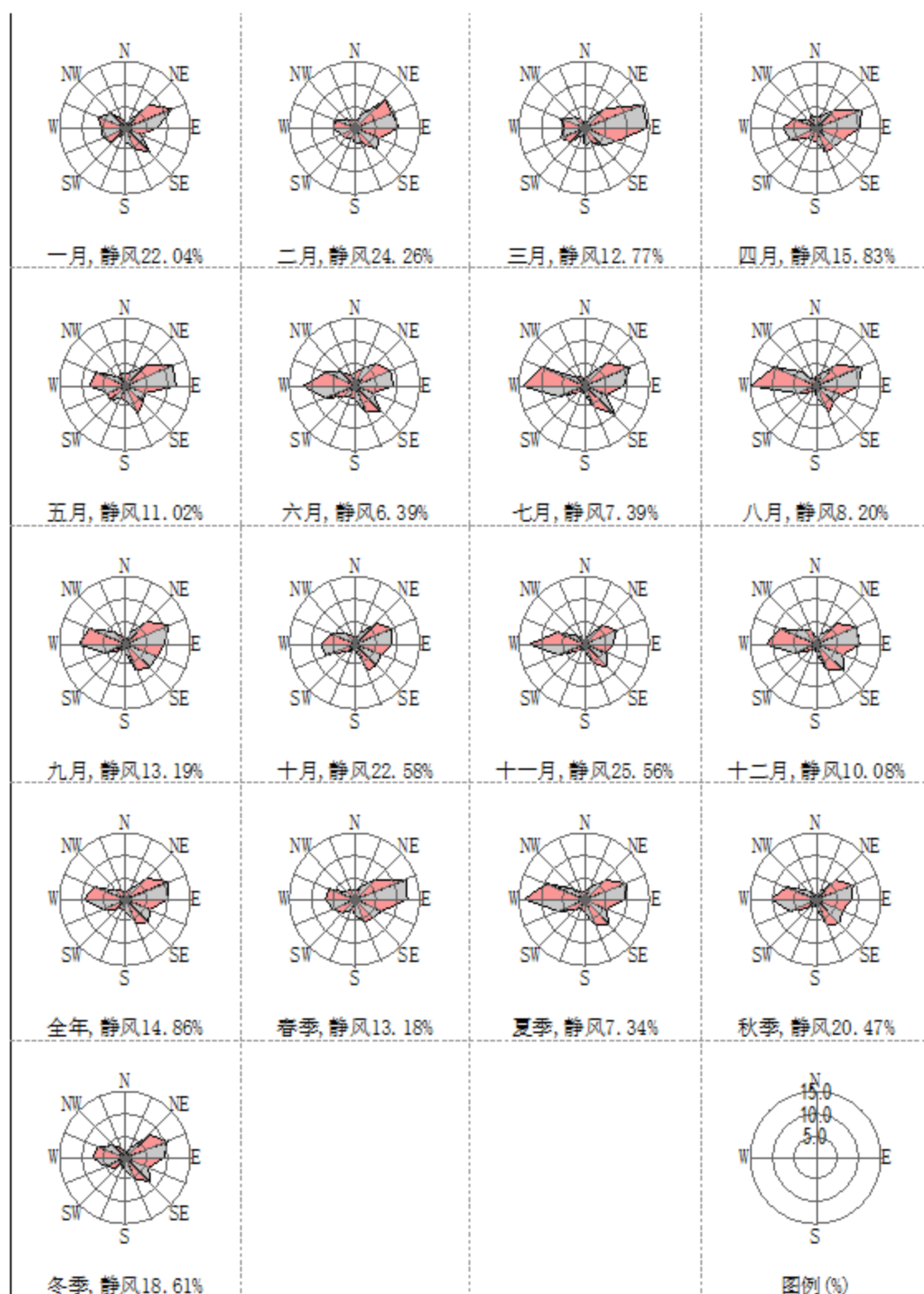
图 5.2.1-1 2024 年风向频率玫瑰图
