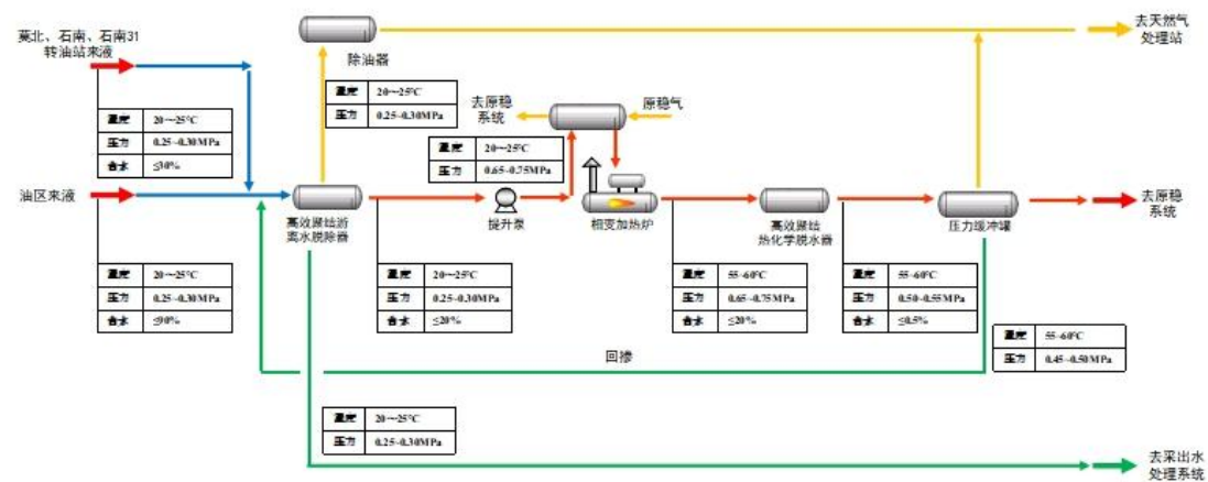
图 3.6-9 石西集中处理站处理工艺流程框图
