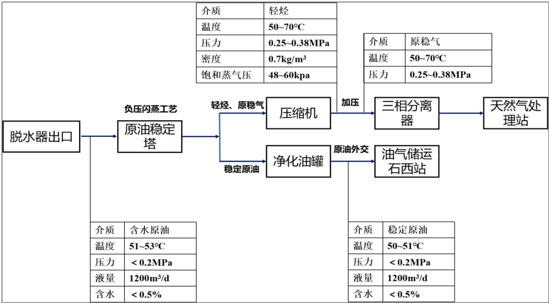
图3.6-10 石西集中处理站原稳工艺流程图
