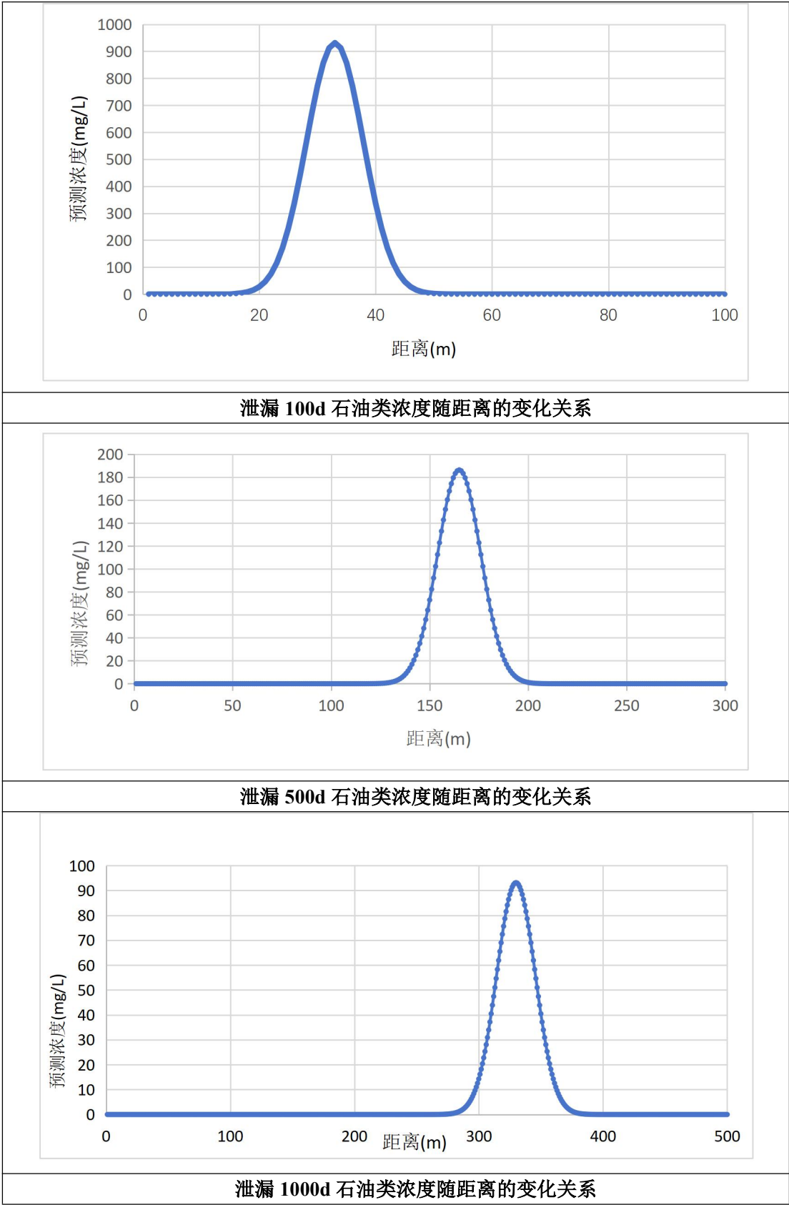
图5.2-3集输管线发生全管径泄漏时石油类浓度随距离的变化关系
