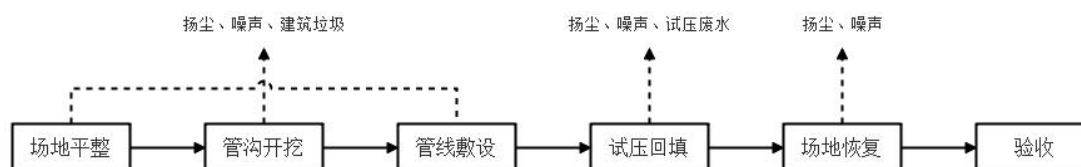
图 3.8-5 集输工程建设工艺流程及产污环节示意图
