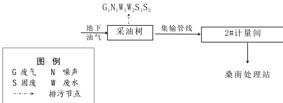
图 3.4-4 井场开采及集输工艺流程图
