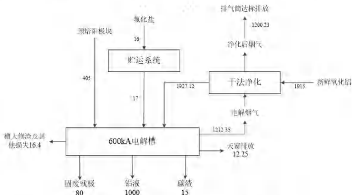
图 3.4-2 电解工序物料平衡图 单位：kg/t-Al
