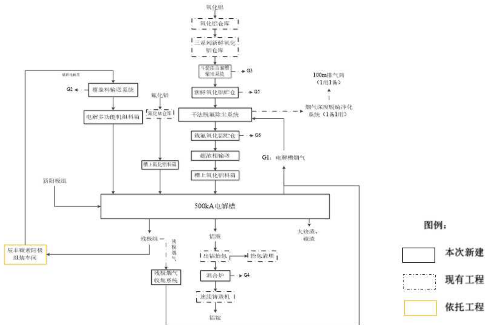
图 3.3-4 项目运营期工艺流程及产污环节图
