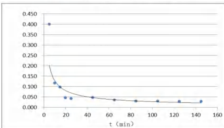
图 5.4-6 厂区中部 sh2 渗水试验曲线图
