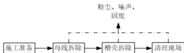
图 3.3-2 二系列电解铝拆除工艺流程及产污节点示意图
