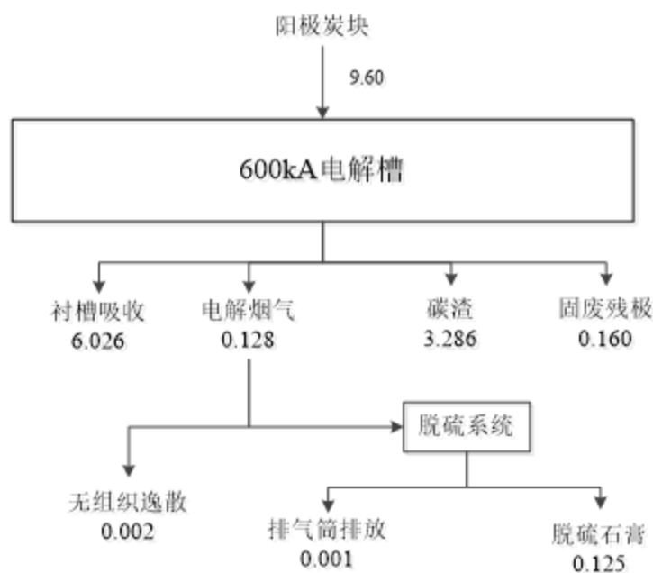
图 3.4-4 氟平衡图 单位: kg/t-Al
