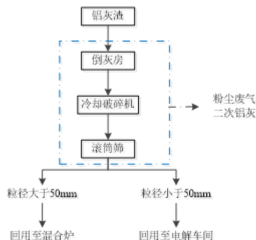
图 3.1-2 铝灰筛分冷却系统工艺流程和产污节点图
