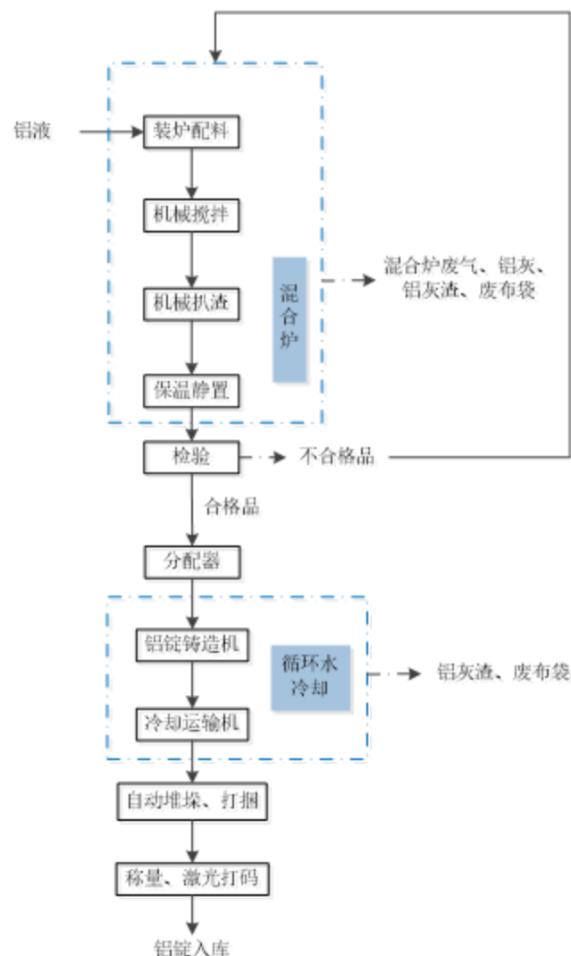
图 3.1-1 铝锭工艺流程和产污节点图
