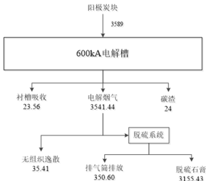
图 3.4-3 硫平衡一览表 单位：t/a
