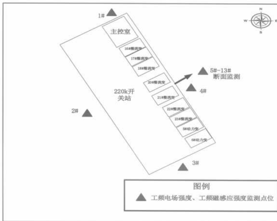
图 5.11-1 类比项目电磁辐射监测布点图
