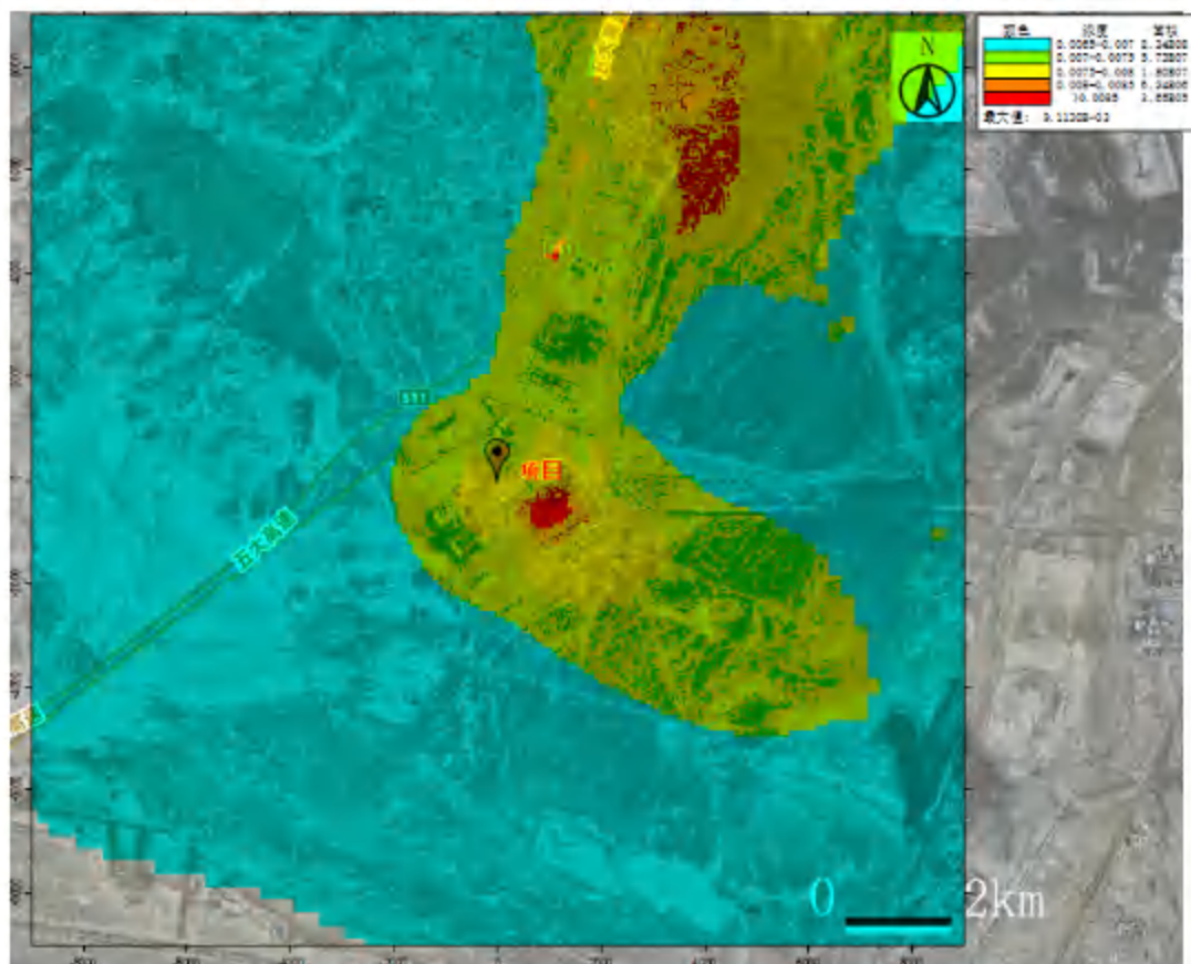
图 5.2-6 网格点 SO 2 保证率日均浓度等值线分布图
