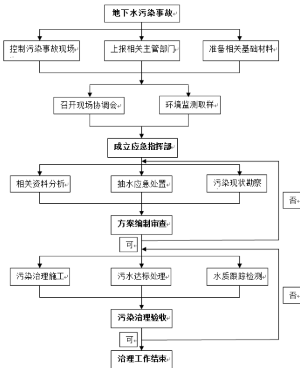
图 6.4-1 地下水污染应急治理程序框图
