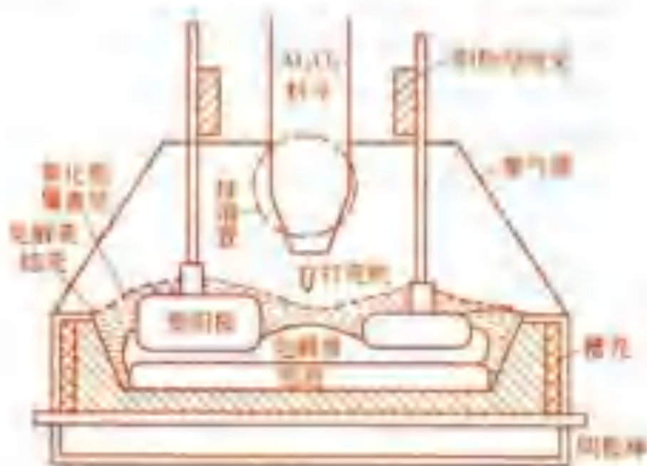
图 3.3-3 电解槽内部示意图
