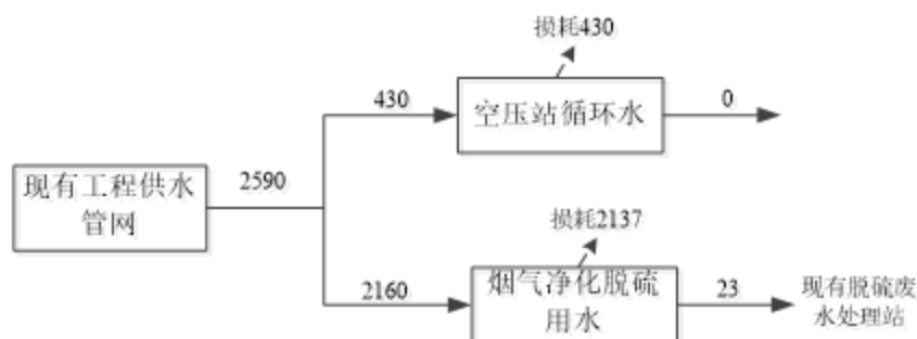
图 3.4-1 项目水平衡图 单位： \text{m}^3/\text{d}
