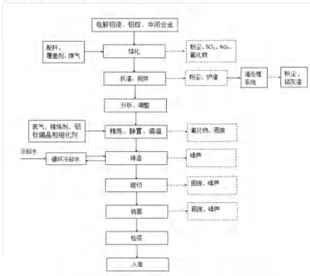
图 3.1-3 铝棒生产工艺流程及产污示意图
