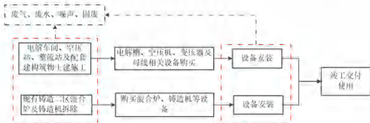
图 3.3-1 拟建内容施工工艺流程及产污节点示意图
