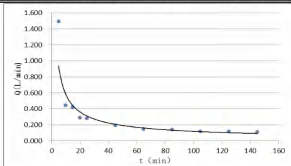
图 5.4-5 厂区北侧 sh1 渗水试验曲线图
