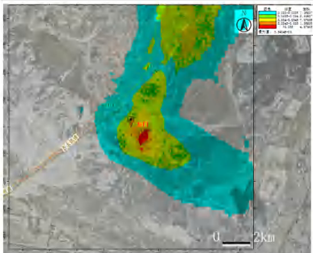
图 5.2-11 网格点本项目叠加拟建项目 PM_{2.5} 年均浓度等值线分布图
