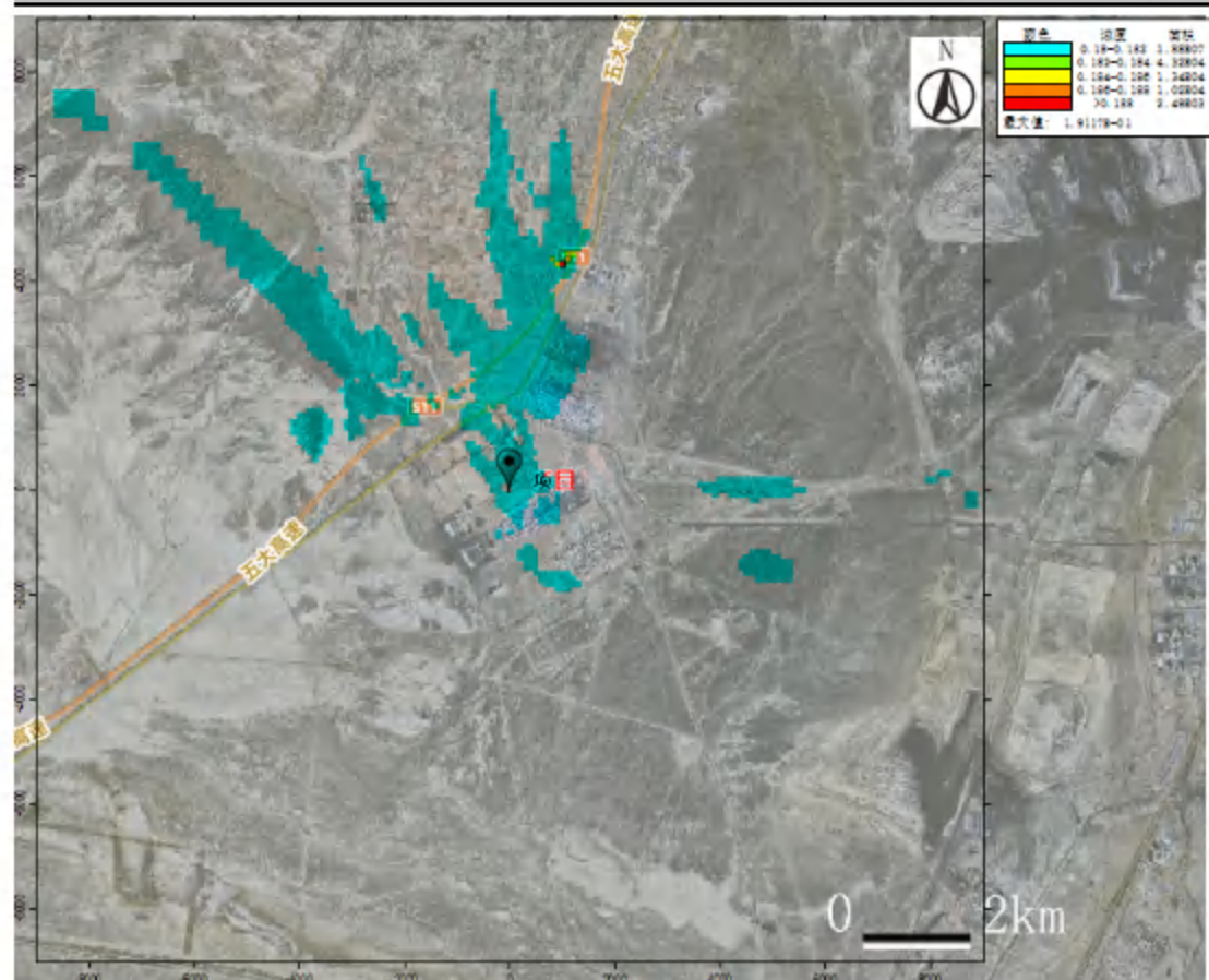
图 5.2-8 网格点本项目叠加拟建项目 PM_{10} 保证率日均浓度值等值线分布图
