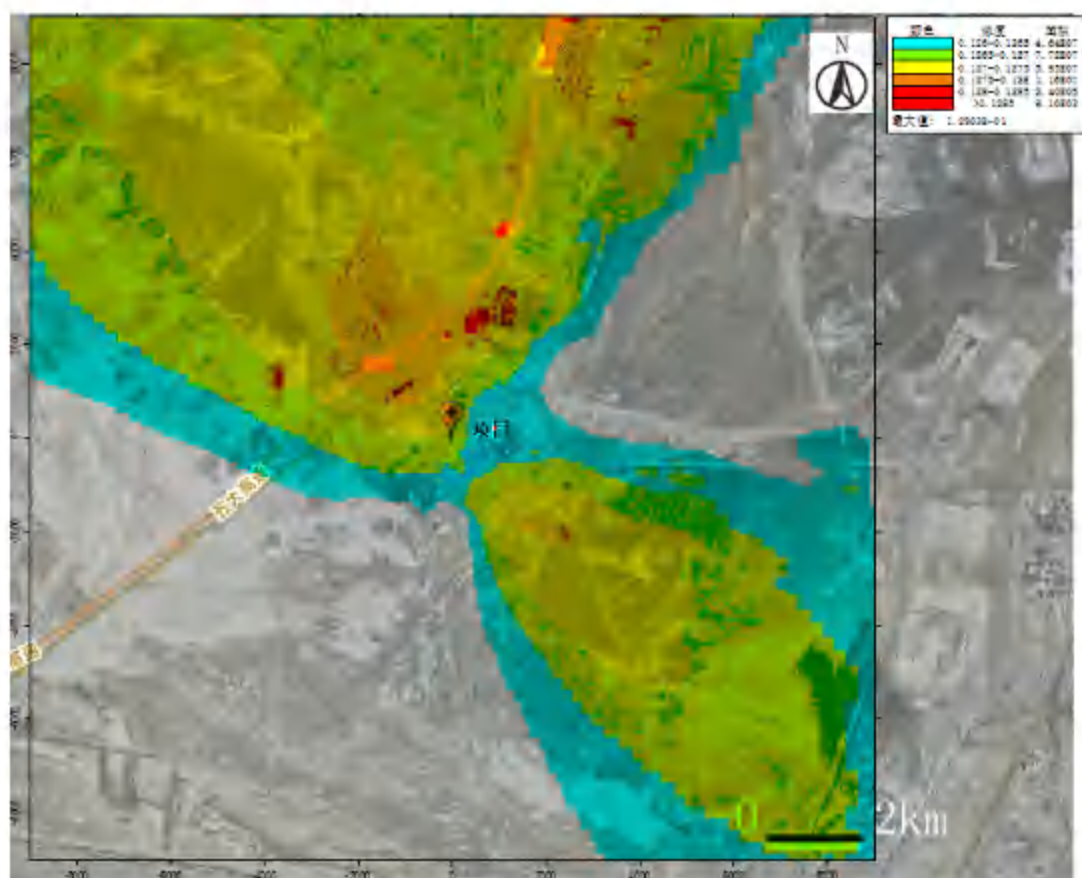
图 5.2-10 网格点本项目叠加拟建项目 \text{PM}_{2.5} 保证率日均浓度值等值线分布图
