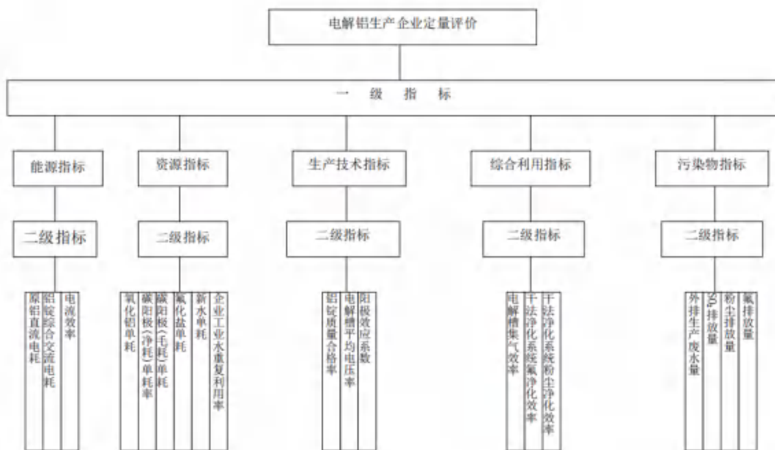
图 3.9-1 电解铝生产企业定量评价框架图
