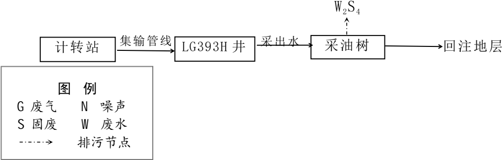
图 3.5-1 注水井场工艺流程图
