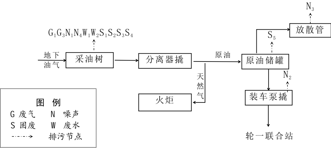
图 3.5-2 台 3 井场开采及集输工艺流程图
