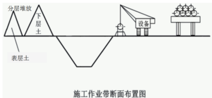
图 3.4-4 一般地段管道施工方式断面示意图
