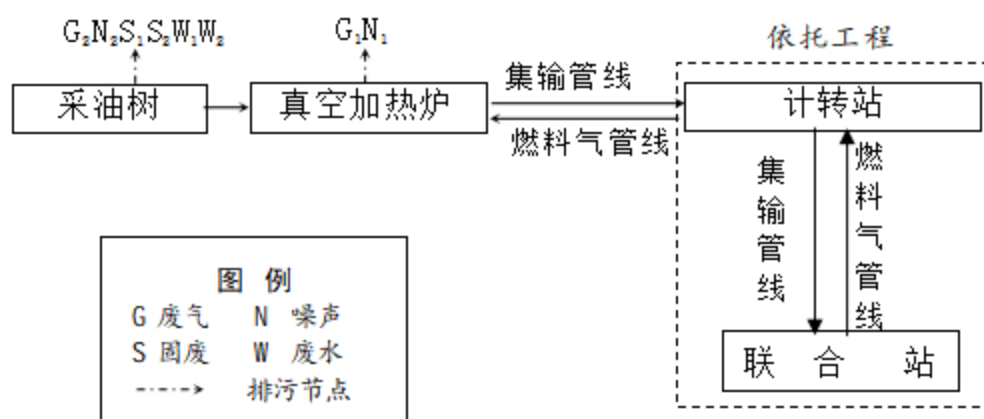
图 3.4-5 新建井场油气开采及集输工艺流程图
