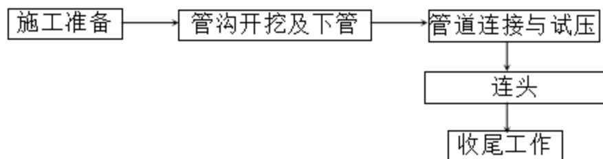
图3.4-3 施工阶段工艺流程图
