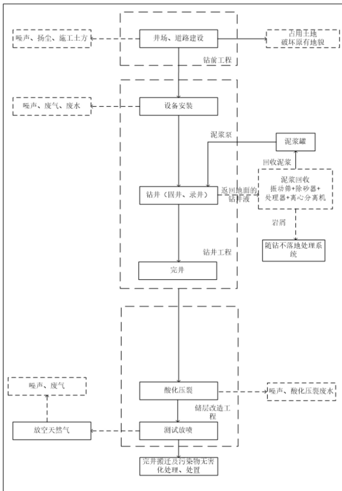
图 3.4-2 钻前工程、钻井工程及储层改造工程工艺流程及污染物排放示意图
